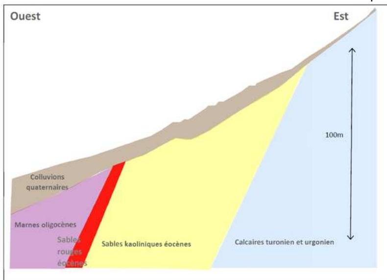
Figure 57 - Coupe géologique schématisée du gisement de sables kaoliniques au nord-ouest de l'anticlinal de Saint-Nazaire (série normale) (source : BRGM RP-70630 provisoire, mars 2021)
