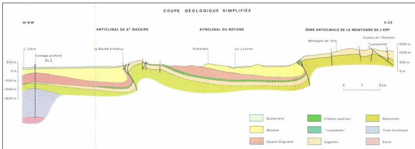
Figure 56 - Coupe géologique simplifiée (carte BRGM 1/50 000 ème ) montrant le gisement kaolinisé à l'ouest de l'anticlinal de St Nazaire et le gisement feldspathique à l'est. (source : BRGM RP-70630 provisoire, mars 2021)
