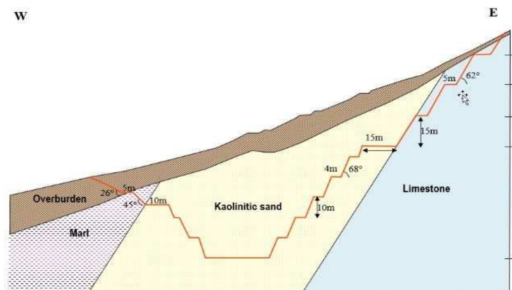
Figure 58 -Vue en coupe du gisement de kaolinite qui montre le débordement de l'exploitation en gradins de part et d'autre des 'épointes' du gisement.(source :BRGM RP-70630 provisoire, mars 2021)
