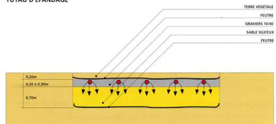
COUPE TRANSVERSALE
