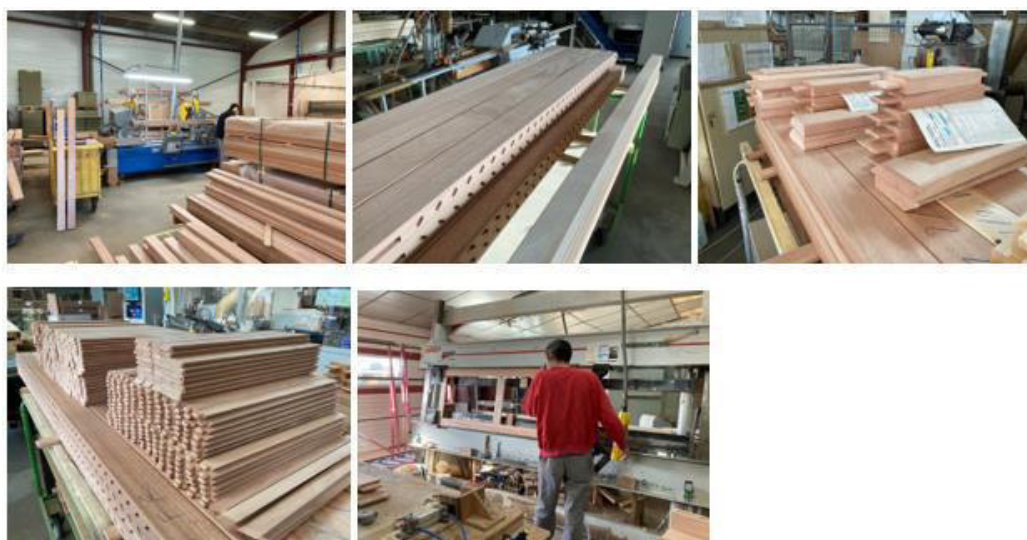
Figure 4 : Ligne de production actuelle, flux volets. De gauche à droite : préparation de profils ; usinages des profils ; assemblage et finition
