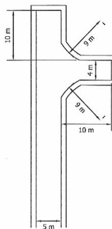
Raquette en Y
