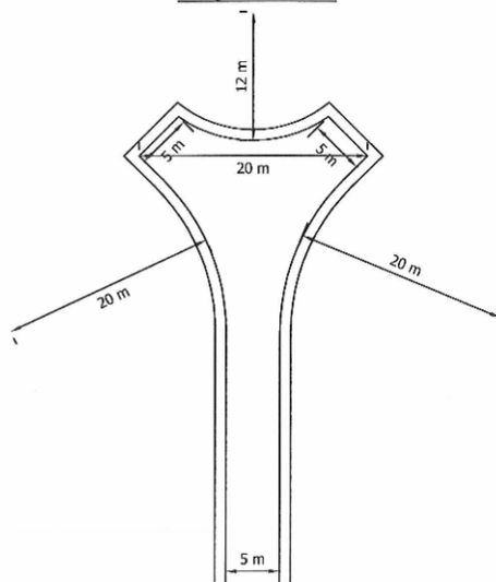
Raquette en Y
