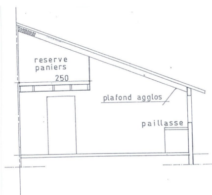
COUPE
