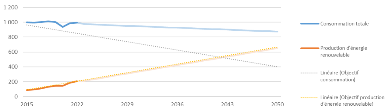
Evolution tendancielle de la production d'énergies renouvelables et de la consommation du territoire en rapport avec les objectifs du PCAET
