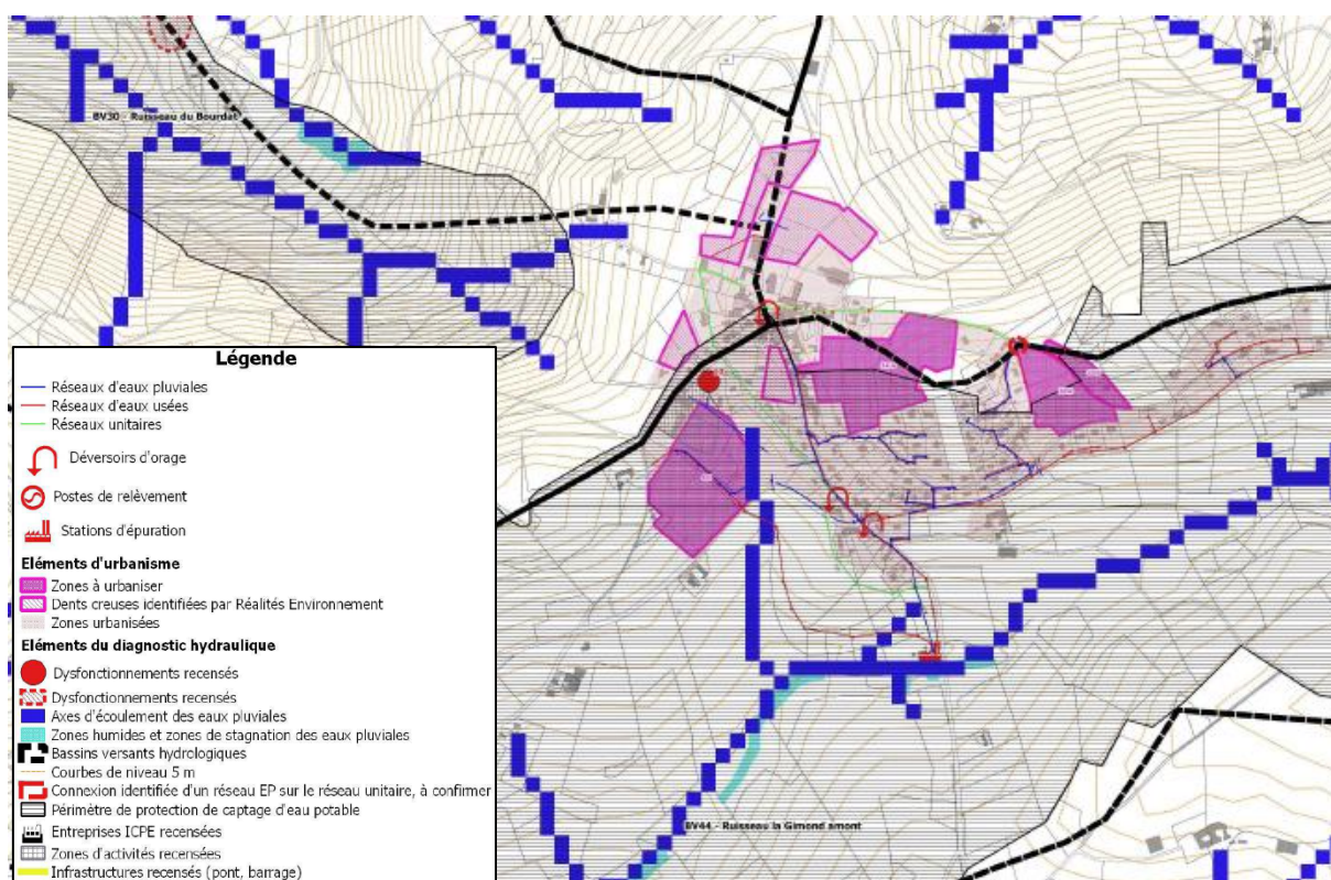
Extrait de la carte de synthèse des contraintes hydrauliques
