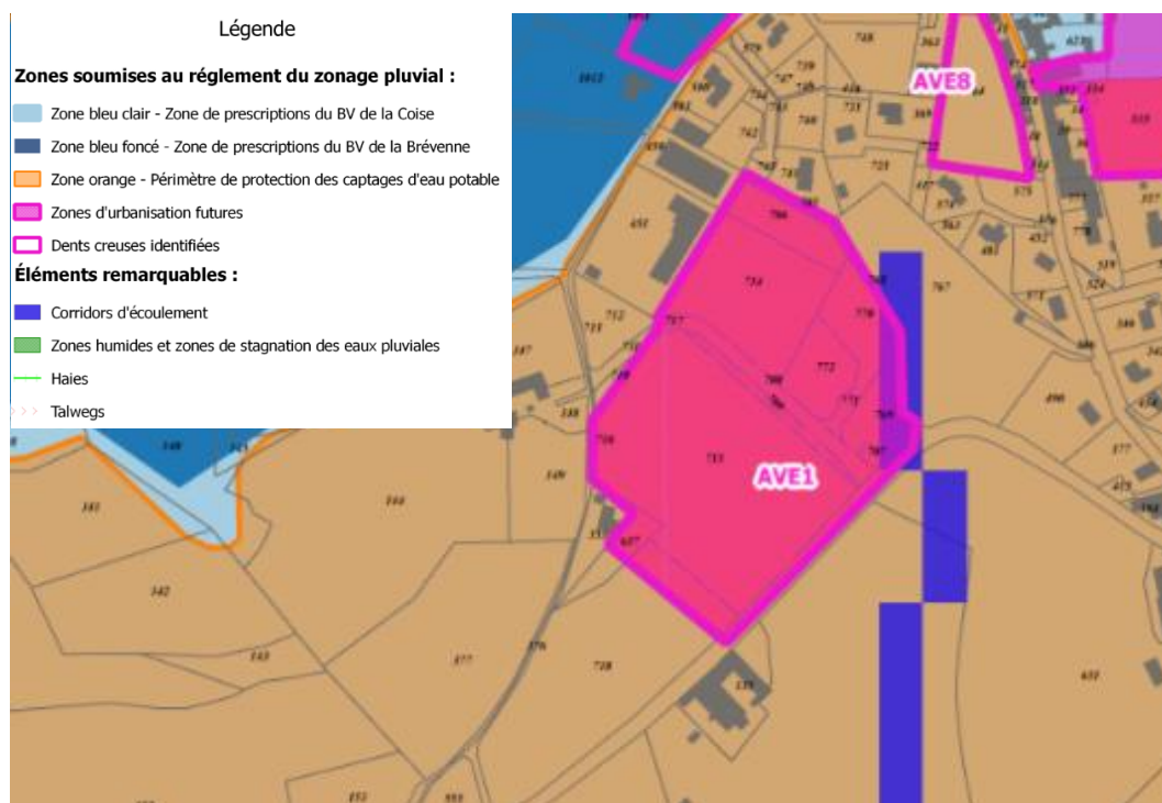
Extrait du plan de zonage des eaux pluviales
