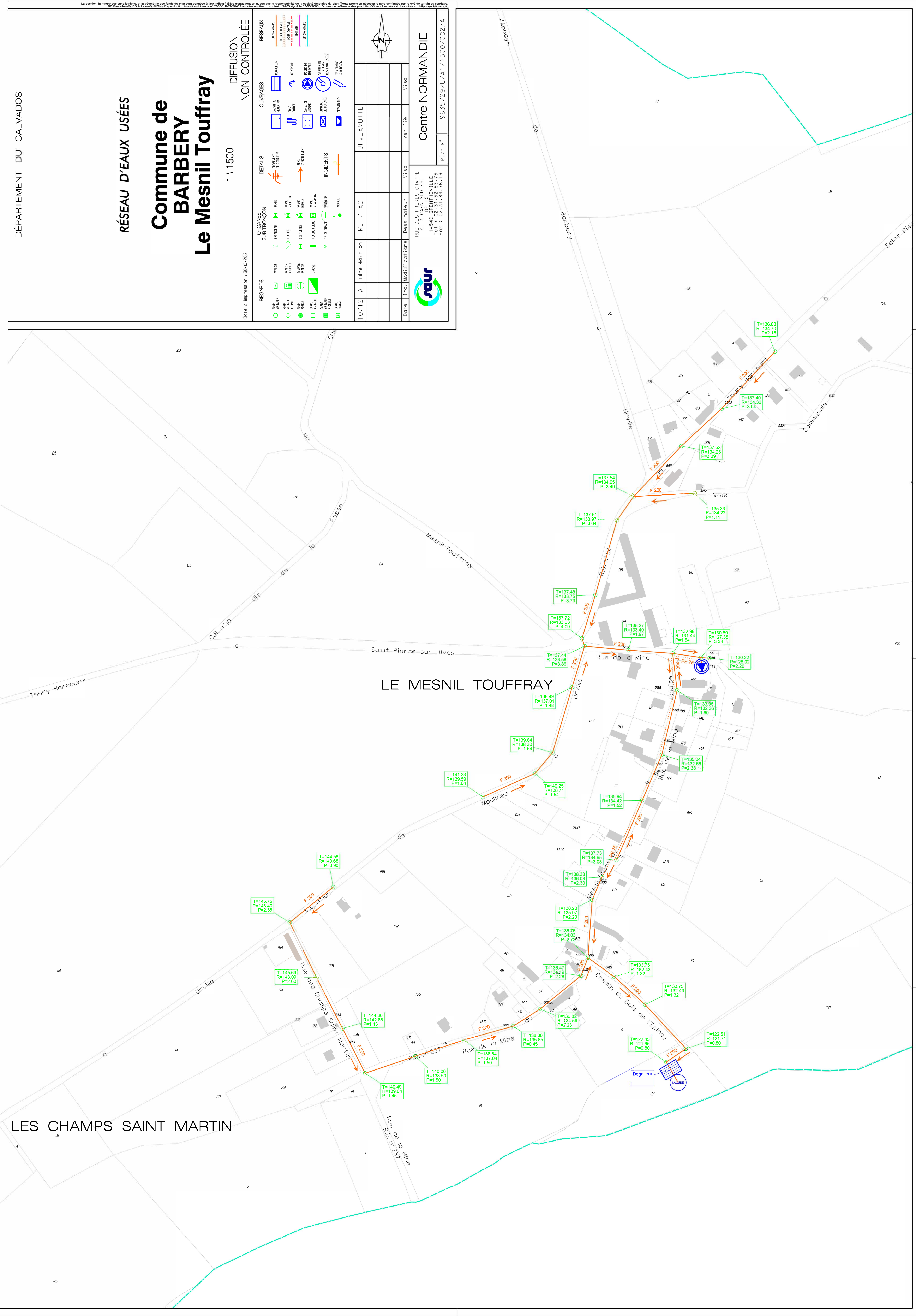
4e2 - RÉSEAUX D'EAUX USÉES - "Le Mesnil Touffray"
