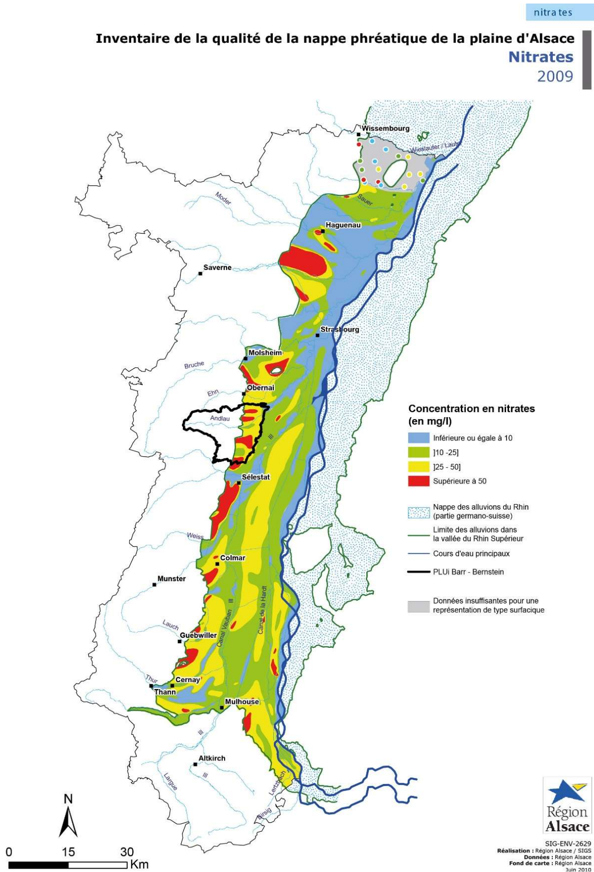
Carte n°5. Inventaire de la qualité de la nappe phréatique de la plaine d'Alsace en 2009
