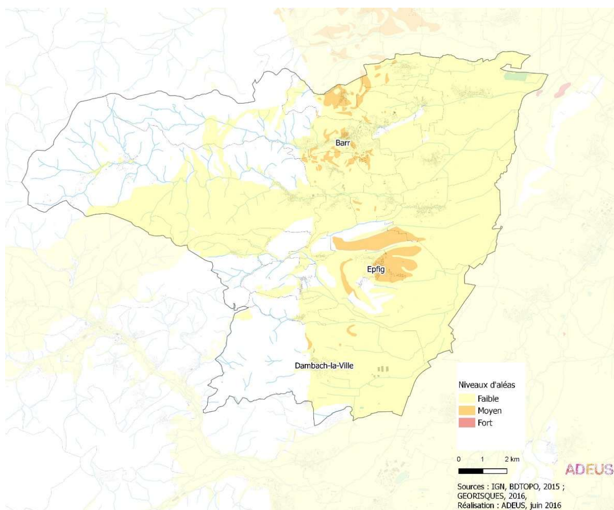
Carte n°9. Aléa retrait gonflement des argiles
