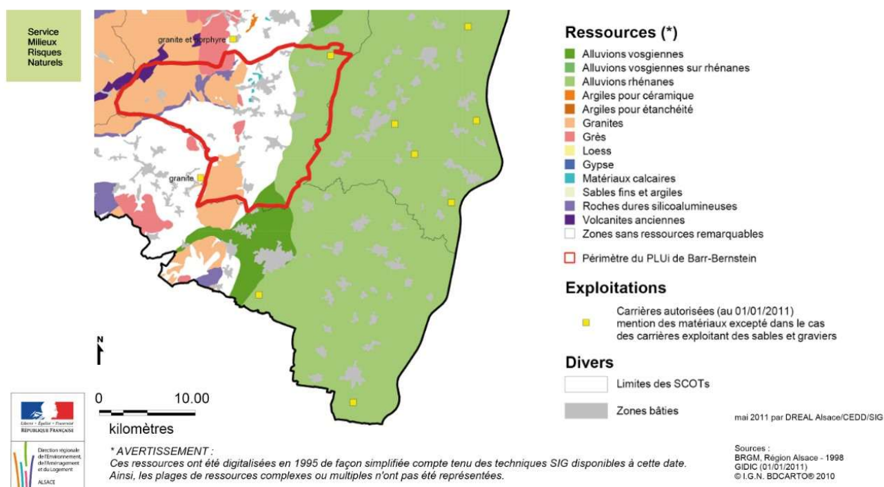
Carte n°12. Zoom de la carte des ressources du Schéma départemental des carrières du Bas-Rhin
