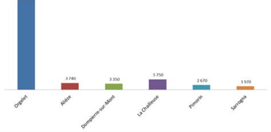
Superficies (ha) impactées par les activités économiques et les équipements collectifs 2006 - 2017 - Soliha IGN
