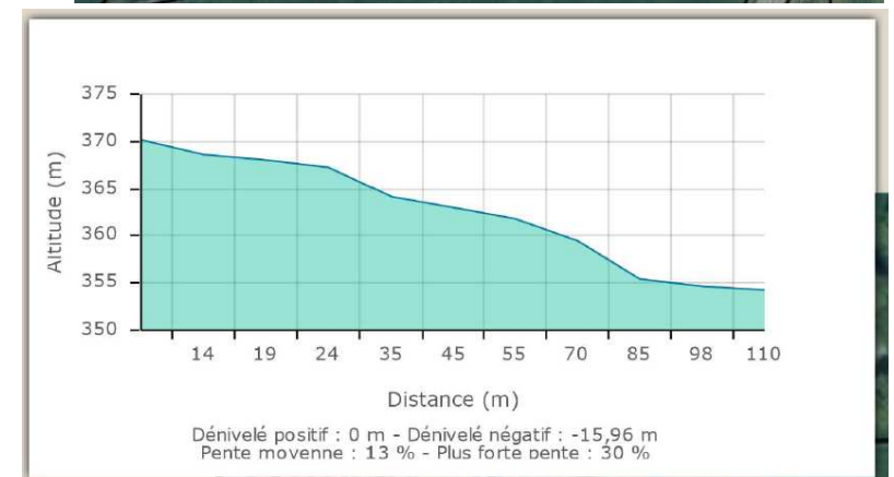
Coupe AA
