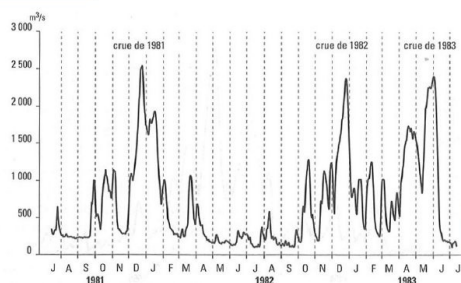
Hydrographes des crues de 1981 82 et 83 à Couzon
