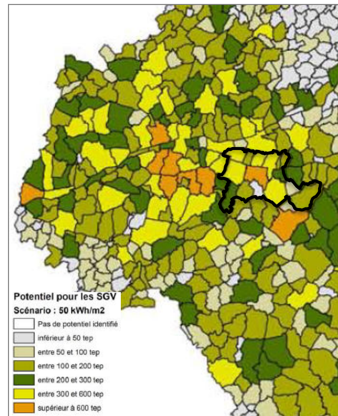
Potentiel géothermique sur sonde géothermique verticale (source : SRCAE Centre, 2012)
