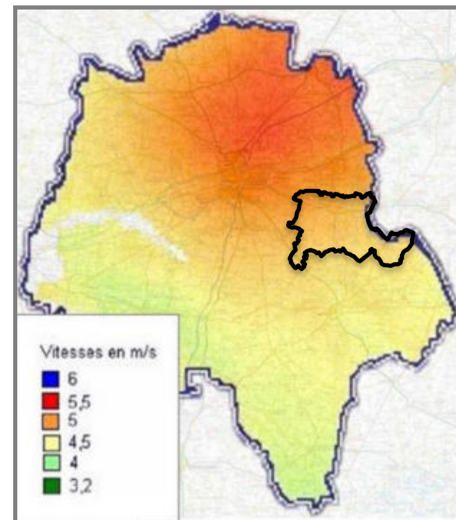
Vitesse moyenne du vent en Indre-et-Loire (source : DREAL Centre-Val de Loire)
