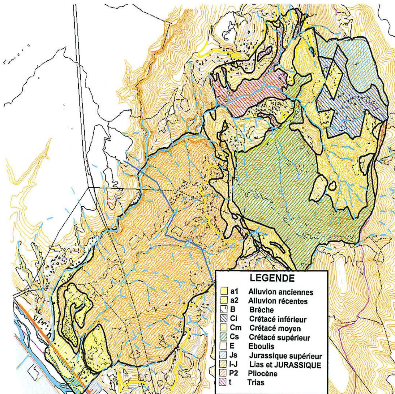
Carte géologique (CETE)
