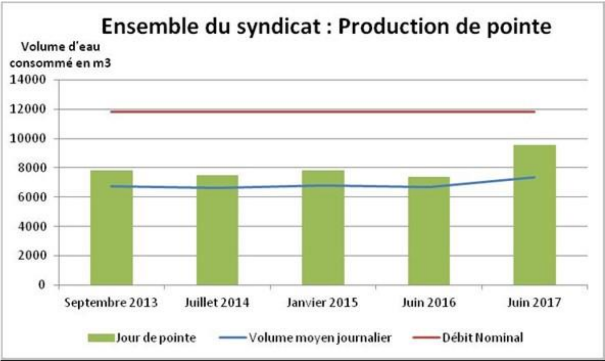
Graphique 13 : Production de pointe
