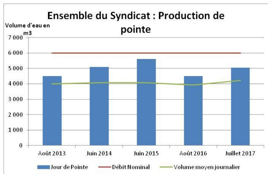
Graphique 15 : Production de pointe SIECSE
