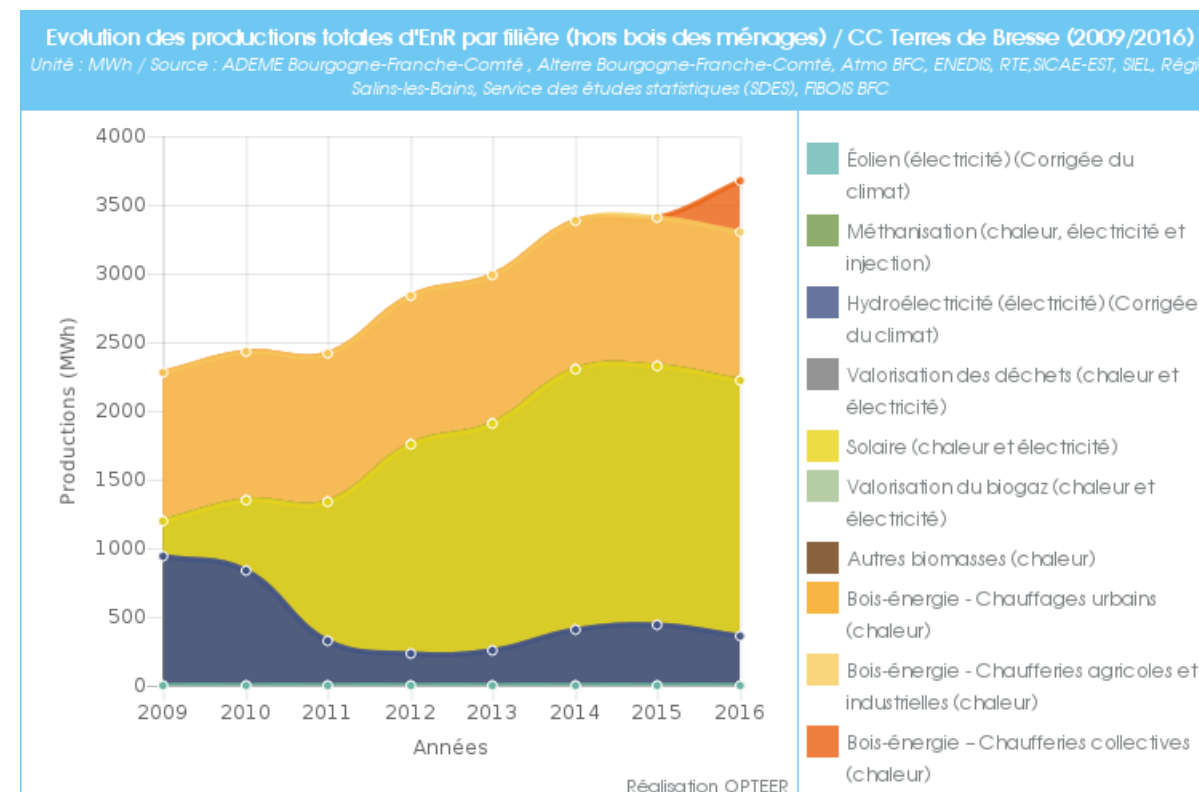
Graphique 26 : Évolution des productions totales d'ENR par filière
