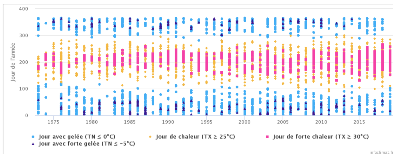
Graphique 4 : Dates des gelées / chaleurs, à Mâcon – Charnay, sur la période 1975 – 2018. Source : Infoclimat.
