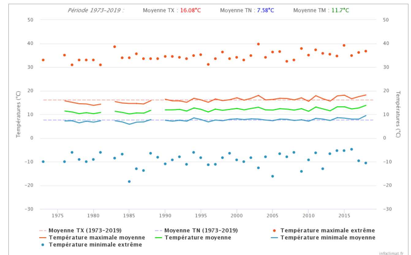
Graphique 2 : Températures (°C) à Mâcon – Charnay, sur la période 1975 – 2018. Source : Infoclimat
