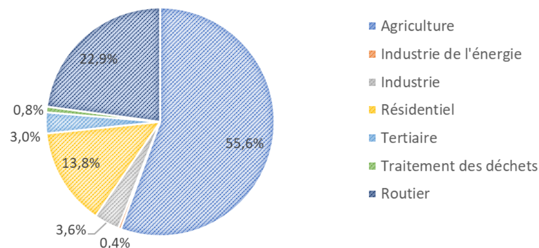
Graphique 27 : Part des différents secteurs dans les émissions de GES, 2014
