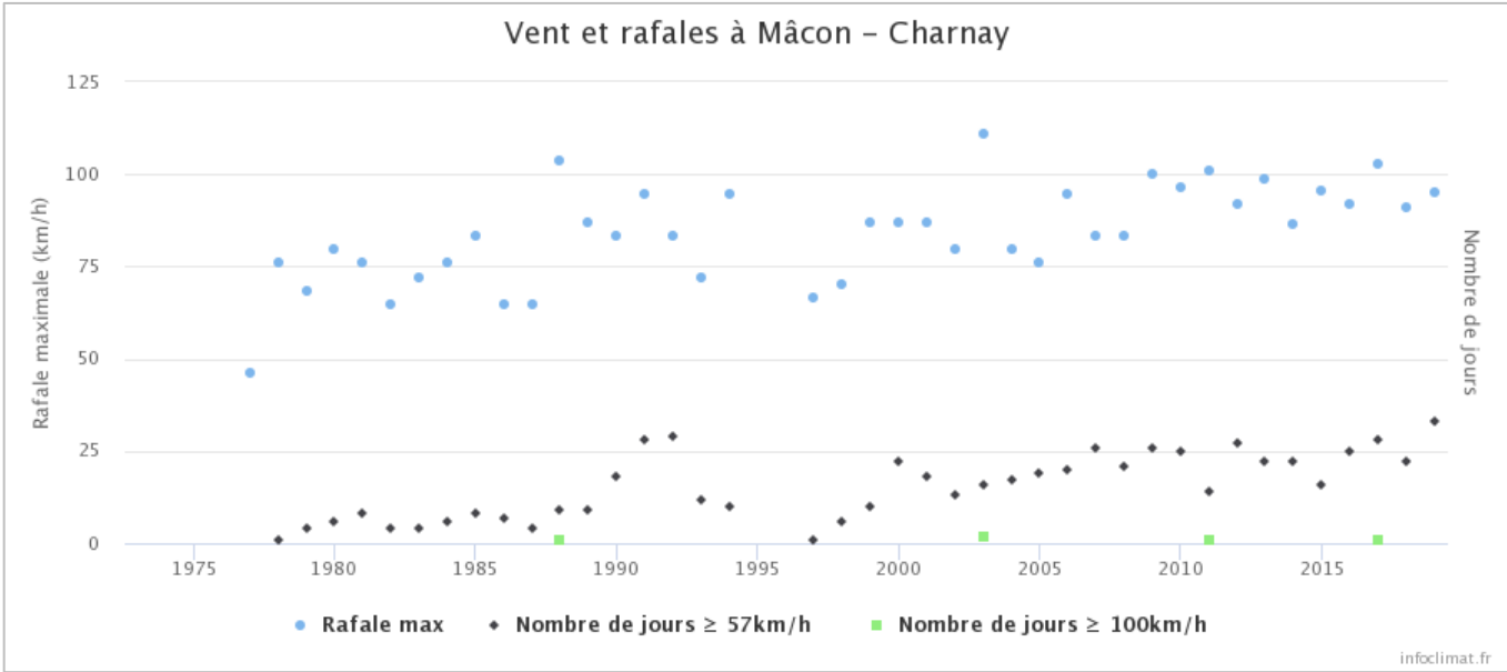
Graphique 9 : Vent et rafales (km/h) à Mâcon – Charnay, sur la période 1975 – 2018. Source : Infoclimat
