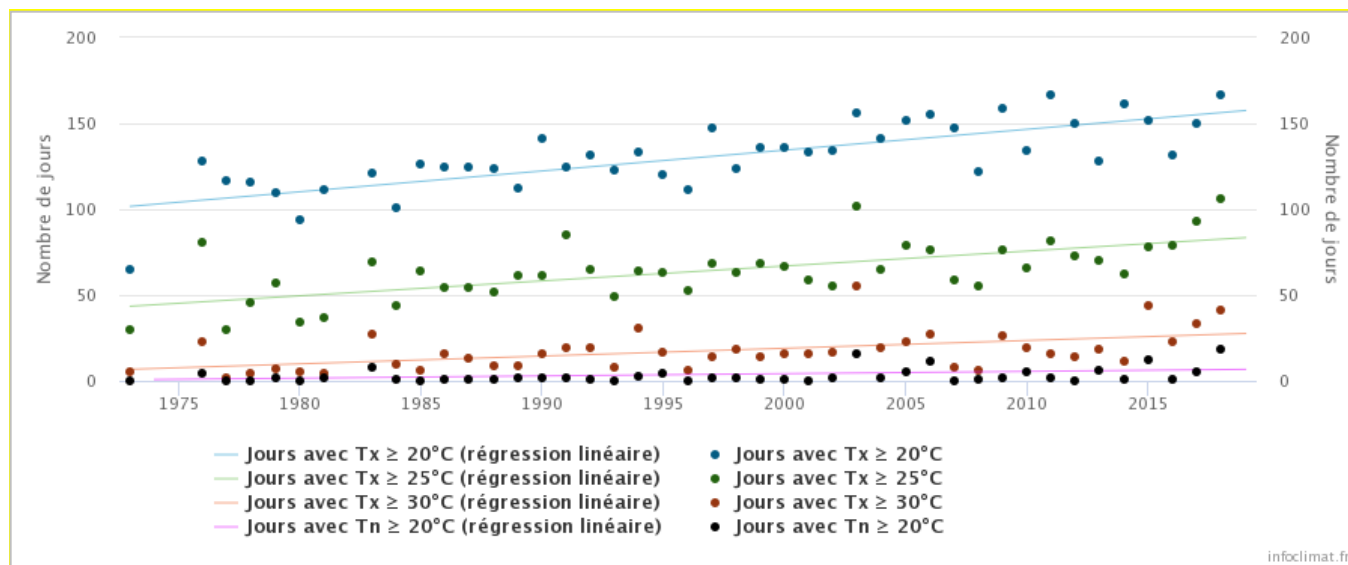
Graphique 3 : Occurrences de chaleur à Mâcon – Charnay, sur la période 1975 – 2018. Source : Infoclimat
