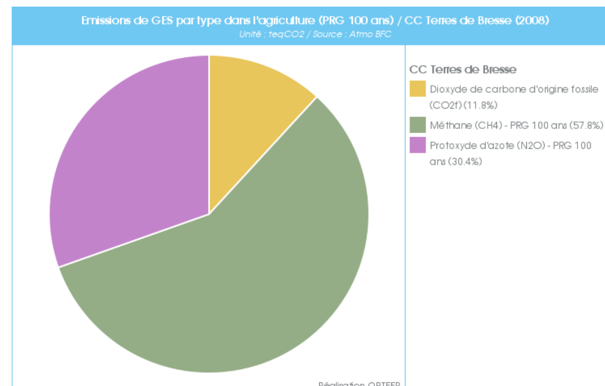
Graphique 28 : Émissions de GES dans l'agriculture, 2008
