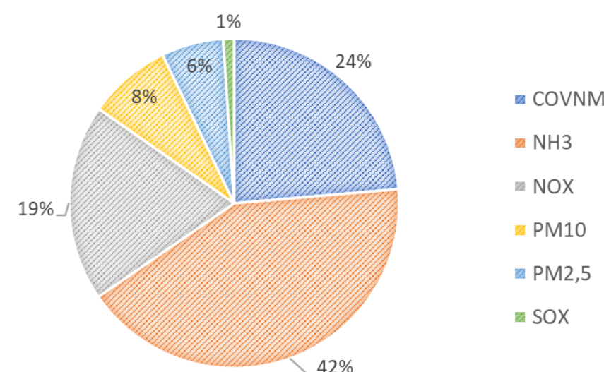
Graphique 20 : Part des polluants dans les émissions de polluants atmosphériques, 2014
