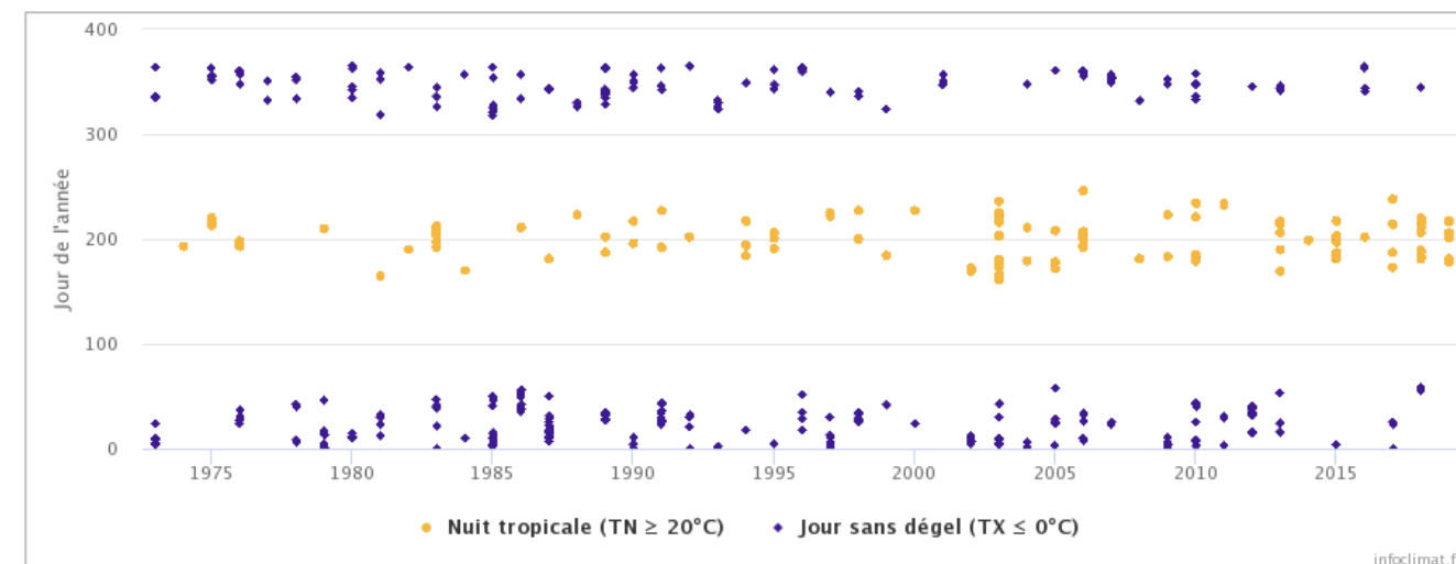
Graphique 5 : Nuits tropicales et journées sans dégel à Mâcon – Charnay, sur la période 1975 – 2018. Source : Infoclimat
