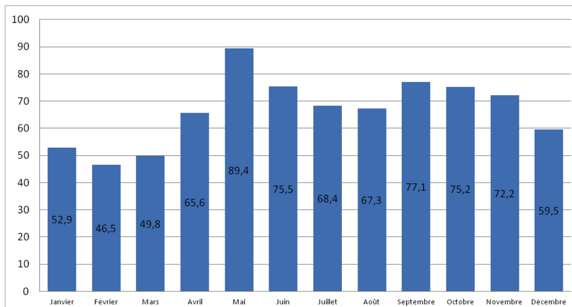
Graphique 6 : Moyenne des précipitations (mm) à Saint-Yan, sur la période 1981 – 2010.
