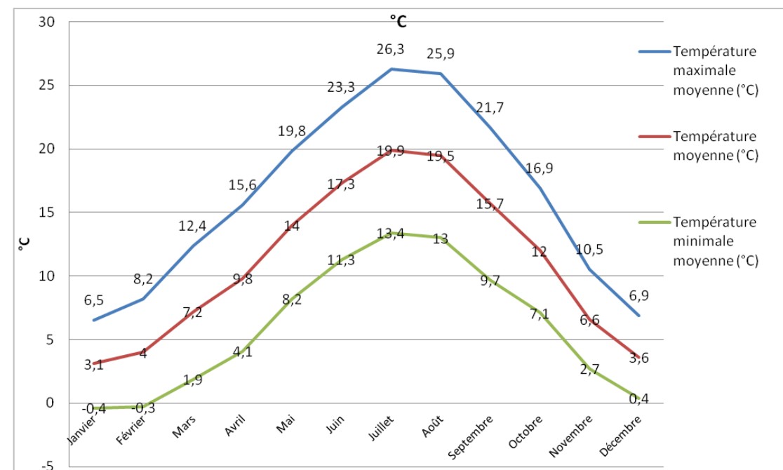
Graphique 1 : Température moyenne (°C), à Saint-Yan, sur la période 1981 - 2010
