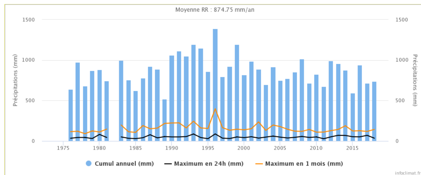
Graphique 7 : Précipitations (mm) à Mâcon – Charnay sur la période 1975 à 2018. Source : Infoclimat
