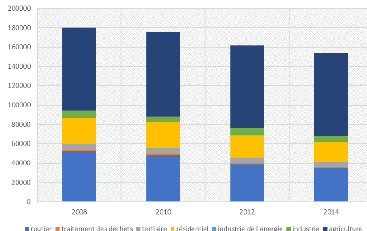
Graphique 29 : Évolution des émissions de GES par secteur 2008-2014
