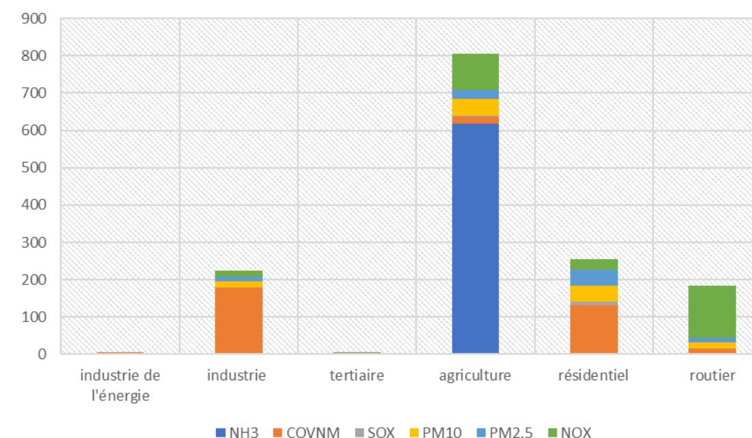
Graphique 21 : Répartition des polluants atmosphériques, par secteur, 2014
