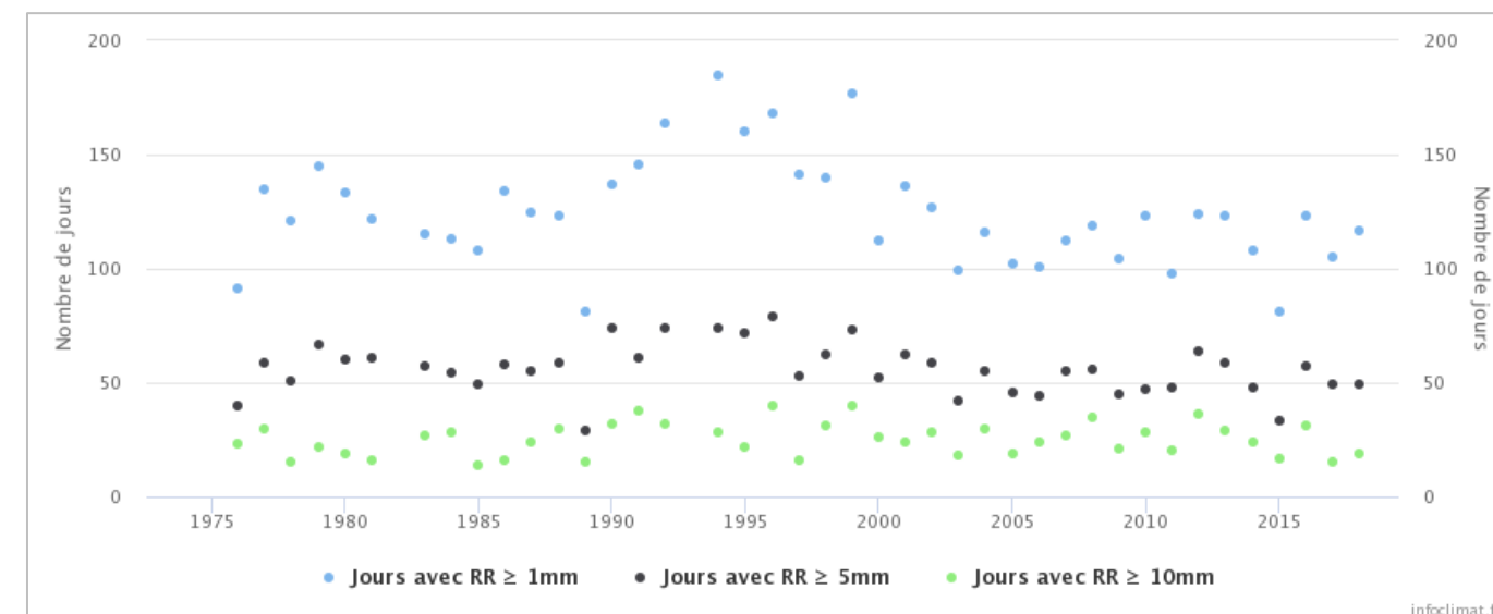
Graphique 8 : Occurrences des précipitations à Mâcon – Charnay, sur la période 1975 à 2018. Source : Infoclimat
