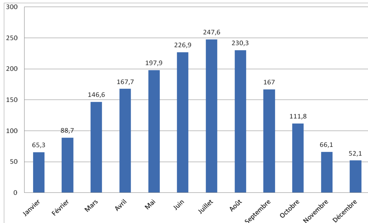
Graphique 11 : Degrés Jours Unifiés (°C) à Saint-Yan, sur la période 1981 – 2010.
