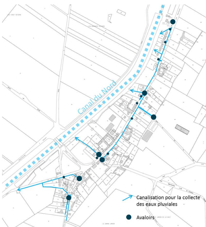
Réseau de collecte des eaux pluviales
