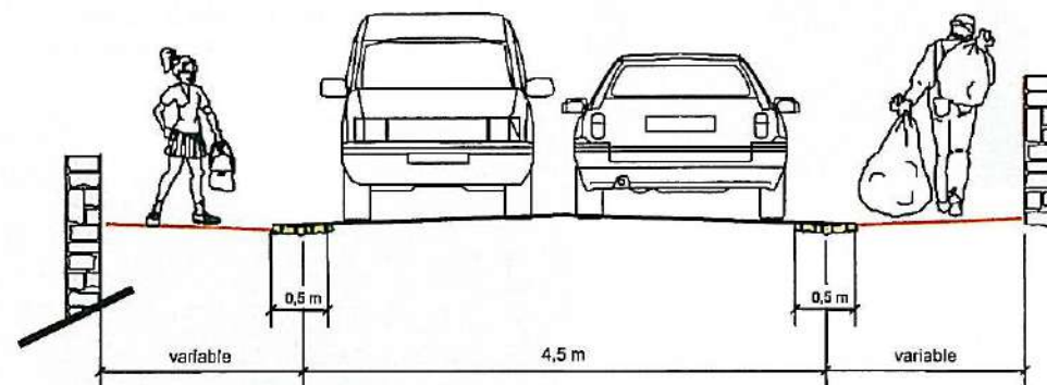
Profil type 2
