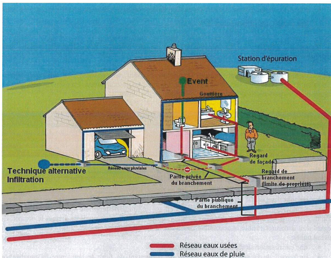
Figure n°3 : Représentation d'un branchement particulier
