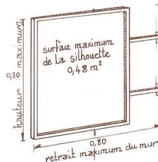
Enseigne drapeau perpendiculaire à la façade
