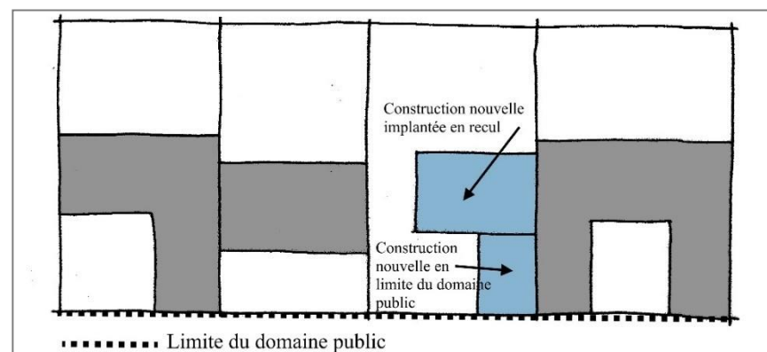
Croquis n°3 : Implantation d'une construction nouvelle en recul du domaine public, prolongée par une construction implantée en « L » à l'alignement du domaine public
