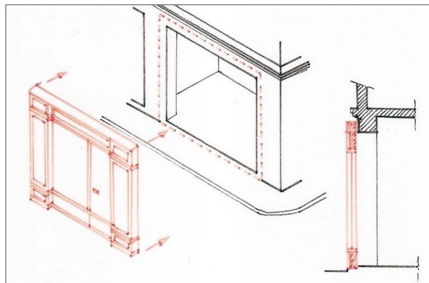
Principe de la devanture en applique
