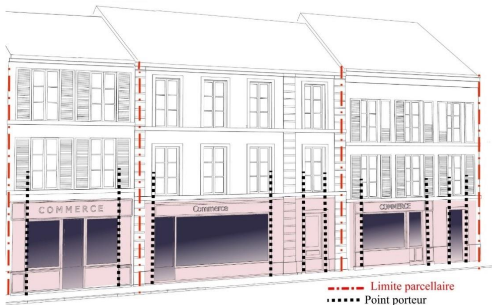
Principe de la devanture en applique
