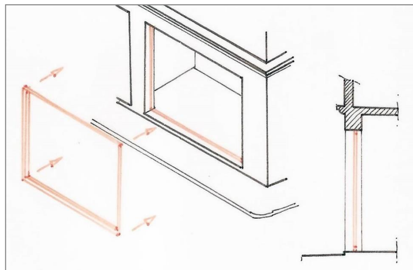
Principe de la vitrine en feuillure
