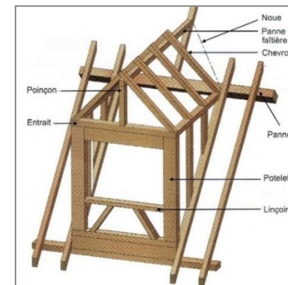
Ossature d'une lucarne charpentée en batière
