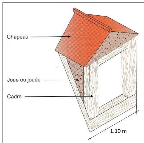
Croquis d'une lucarne charpentée en batière
