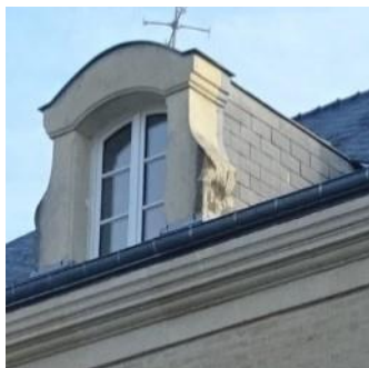
Lucarnes à encadrement de pierre et linteau cintré ou droit
