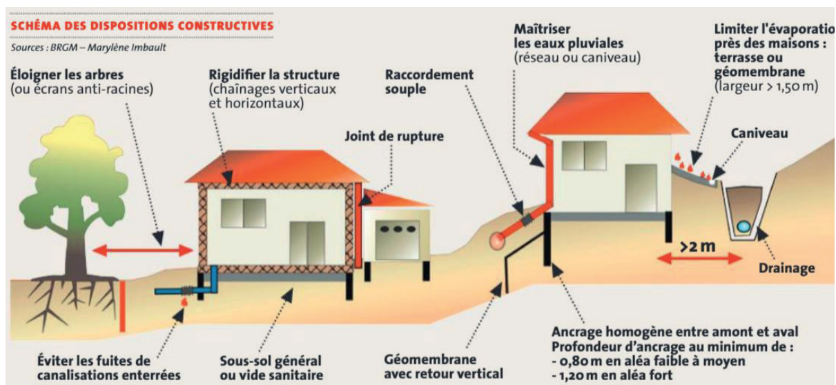
Schéma des dispositions constructives Source : BRGM
