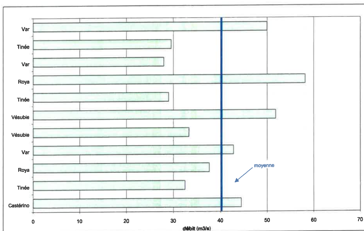
Figure 6 : estimations du débit décennal par analogie
