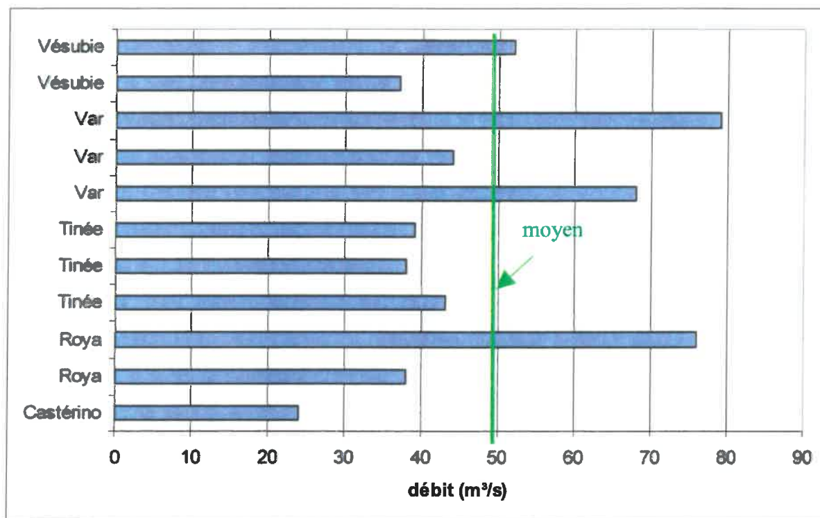
Figure 7 : estimation du débit décennal par analogie
