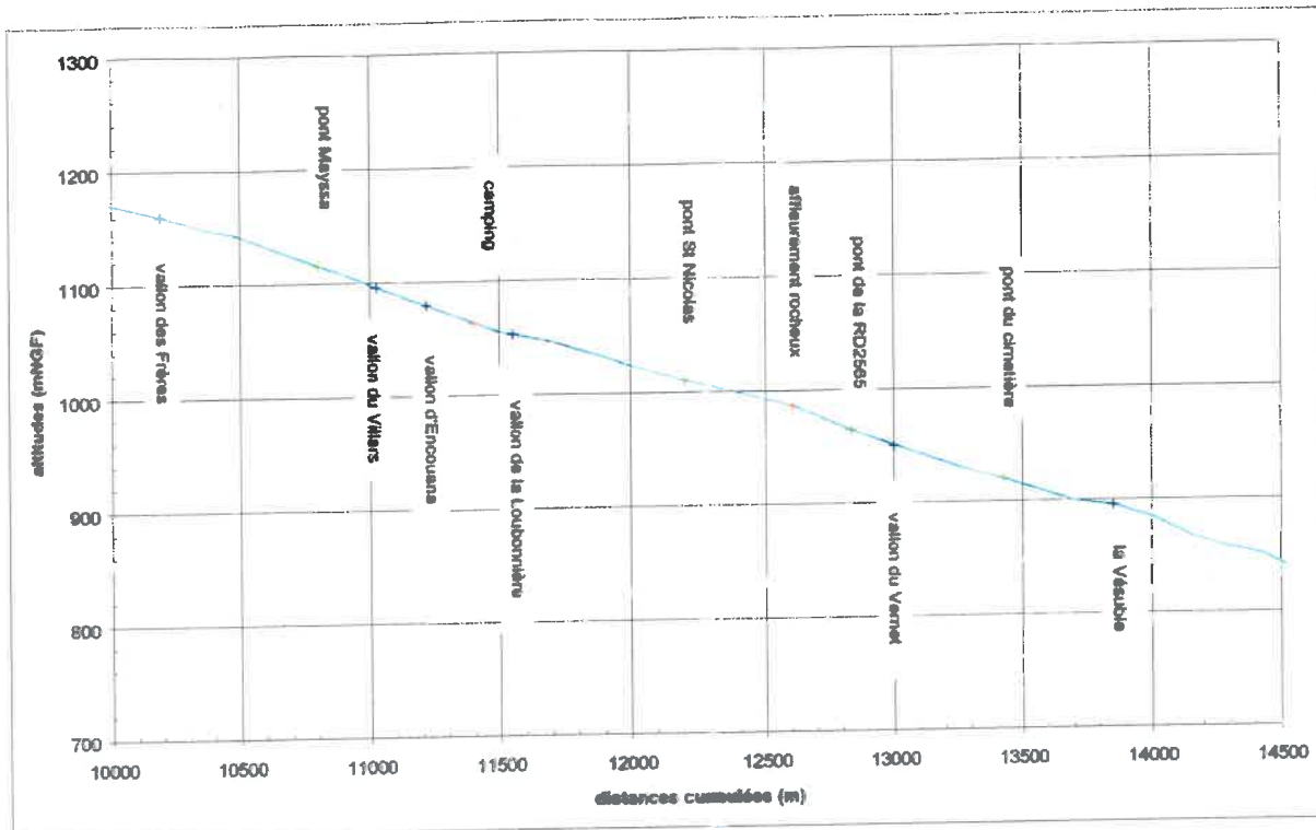
Profil longitudinal du Boréon dans la traversée de Saint Martin Vésubie
