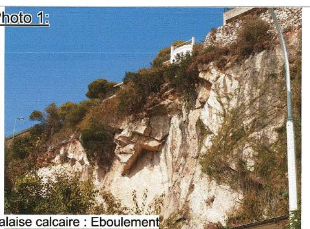
Falaise calcaire - Eboulement
