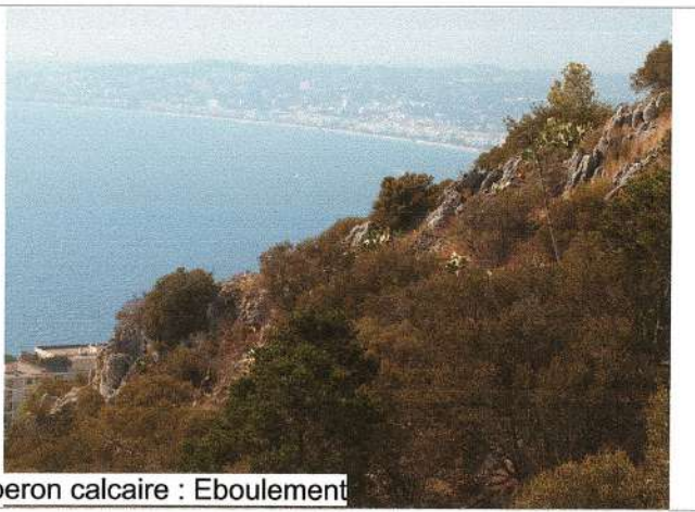
Eperon calcaire - Eboulement
