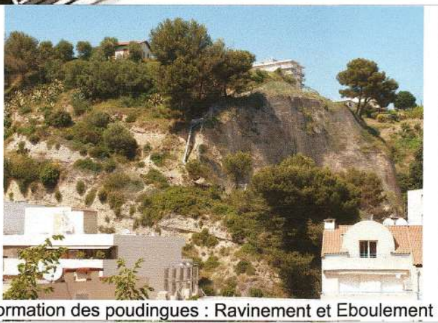
Formation des poudingues : Ravinement et Eboulement
