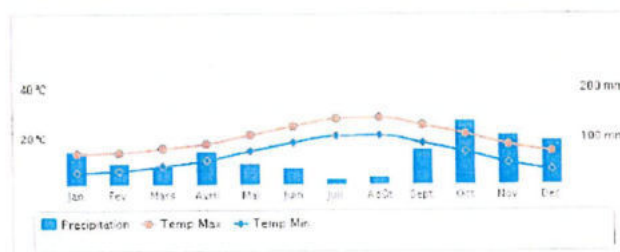
Illustration 3: Moyenne des précipitations (en mm) 1981-2010 Station de Nice (Source Météofrance)
