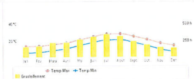
Illustration 2: Moyenne de la durée d'ensoleillement (en h) 1991 - 2010 Station de Nice (Source Météofrance)
