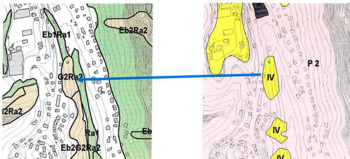
Exemple 1 : limite due à une limite géologique
