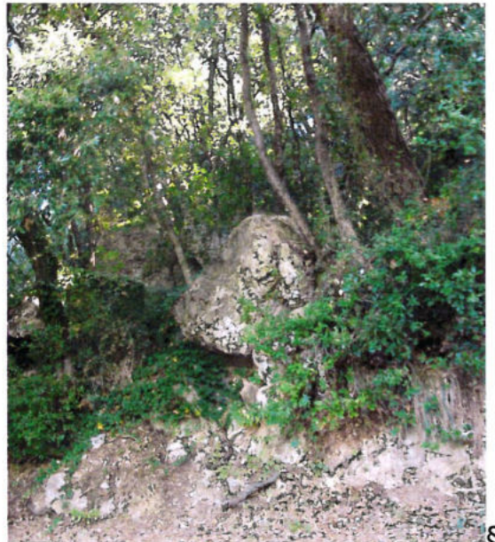
Photo 3 : Ancien bloc éboulé : parc du Mont Vinaigrier
