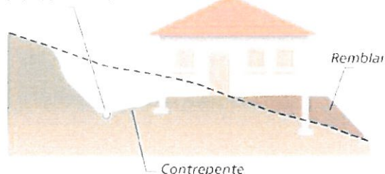
Plate-forme en déblais-remblais
