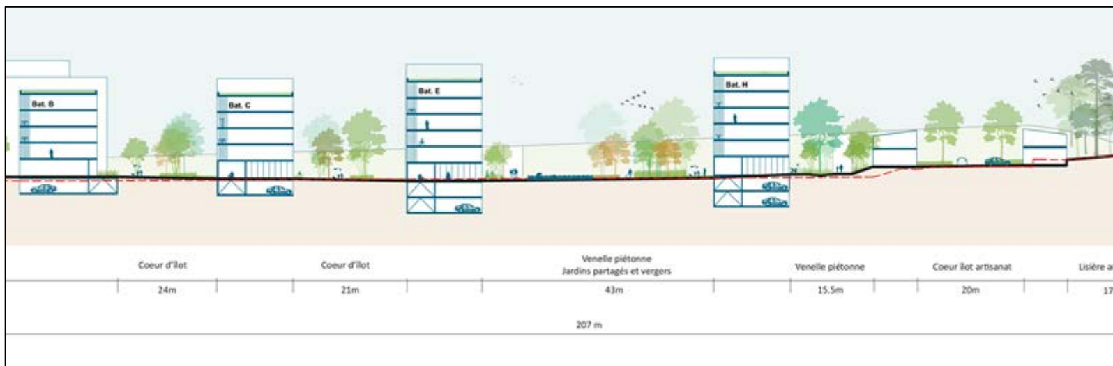
Figure 53 : Coupe Sud-Nord des nouvelles constructions : implantation en peigne, le long de l'avenue de la Sauvegarde
