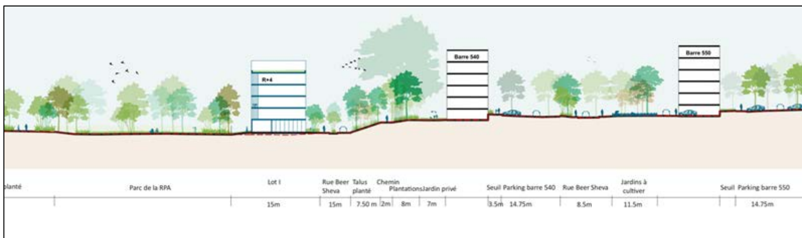
Figure 54 : Coupe Sud-Nord : Implantation de long de la rue Beer Sheva, dans la continuité des réhabilitations des barres 540 et 550
