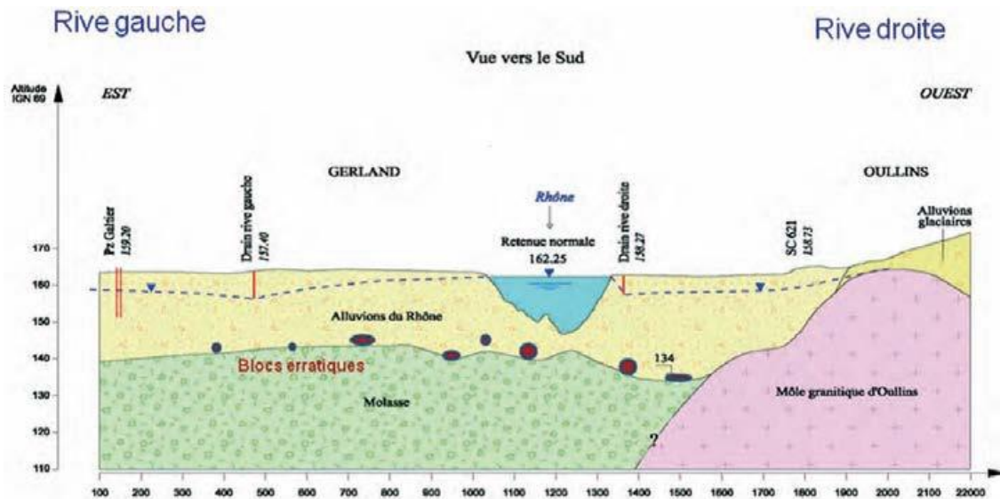
Figure 4 : Extrait de l'étude géologique réalisée dans le cadre de la réalisation du prolongement de la ligne B
