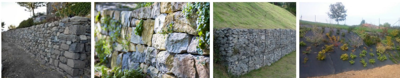
Exemples de traitement des talus : mur de pierres sèches, enrochement, gabion de pierres locales, talus végétalisé
