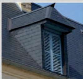
Lucarne «capucine». Sa toiture a 2 pans.
