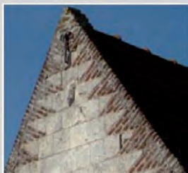
Appareillage «à couteaux». Terminaison haute du pignon qui permet de constituer un angle régulier, ici en brique.
