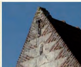
Appareillage «à couteaux». Terminaison haute du pignon qui permet de constituer un angle régulier, en brique ou en brique et moellons de craie.
