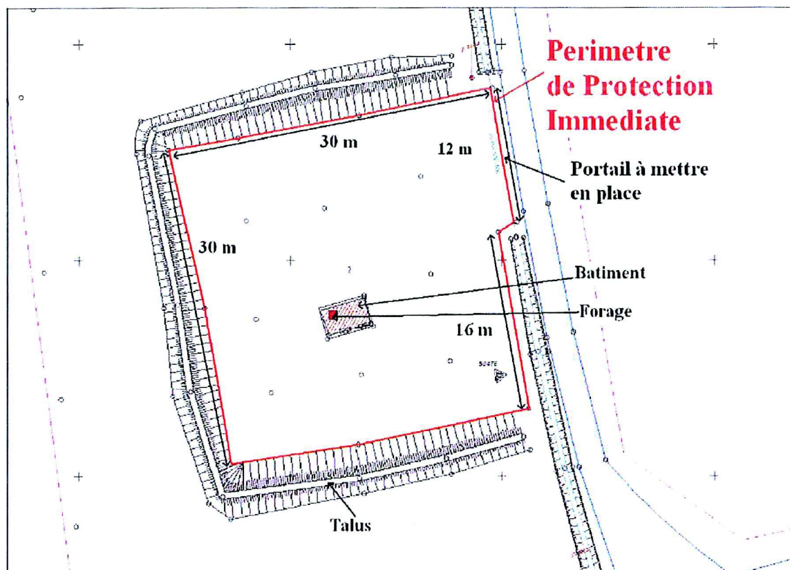
Fraction de la parcelle IZ0024, pleine propriété de la ville de Castres, 1150 m 2
