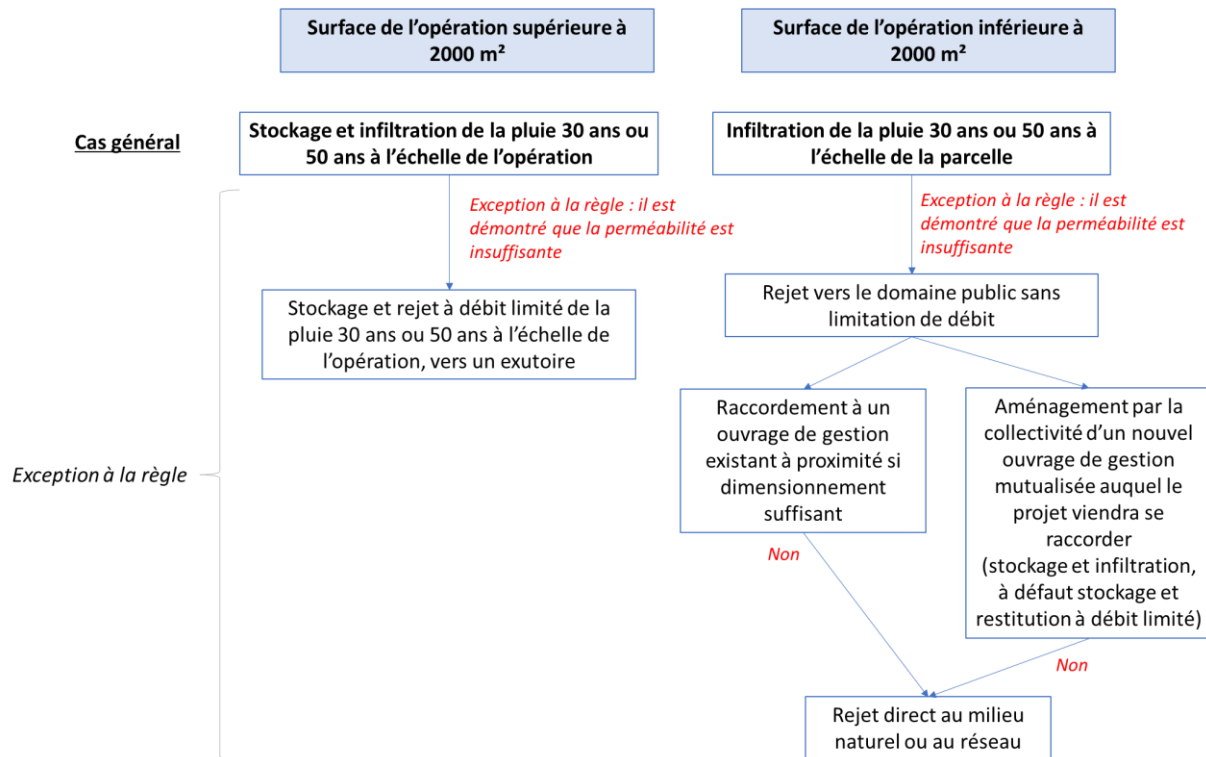
Figure 7 : Logigramme de gestion des pluies moyennes à fortes
