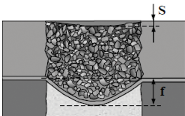
Figure 25 : mise en tension d'une géogridde au-dessus d'une cavité sous l'effet de l'effondrement des terrains sus-jacents (P. Villard, 2006)
