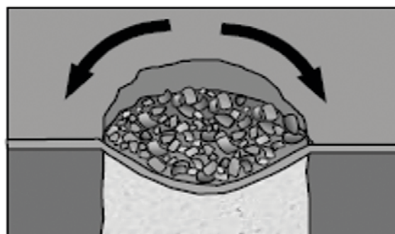
Figure 25 : mise en tension d'une géogridde au-dessus d'une cavité sous l'effet de l'effondrement des terrains sus-jacents (P. Villard, 2006)
