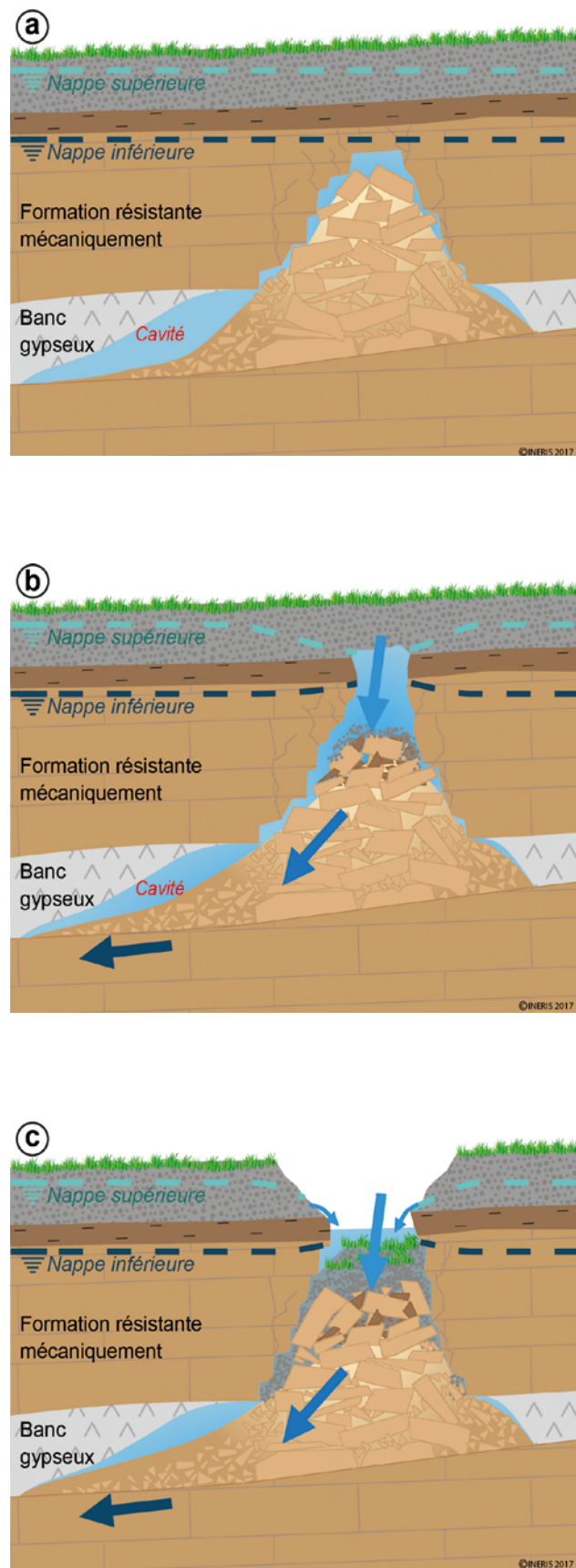
Figure 12 : schémas représentant la propagation du vide jusqu'à la surface par rupture de l'écran imperméable de la nappe sus-jacente. Le vide proche de l'autocomblement (a), continue sa progression vers la surface grâce aux processus d'érosion et de suffosion qui se mettent en place (b et c)
