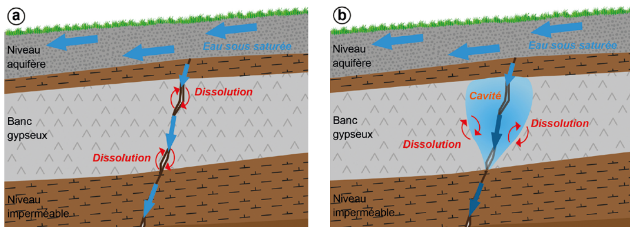
Figure 9 : schéma représentant la mise en place d'un processus de dissolution via une fracture préexistante qui découpe le niveau gypseux. L'eau sous-saturée circule au sein de l'horizon gypseux (ici dans le cas d'une percolation descendante) par l'intermédiaire de la discontinuité (a) et la dissolution peut alors contribuer à la création d'un vide (b)
