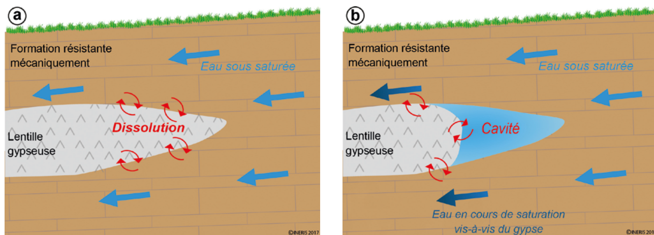
Figure 8 : schéma représentant la mise en place du processus de dissolution au sein d'un aquifère. L'eau sous-saturée en contact avec le gypse (a) entraîne la création de vide par dissolution (b)
