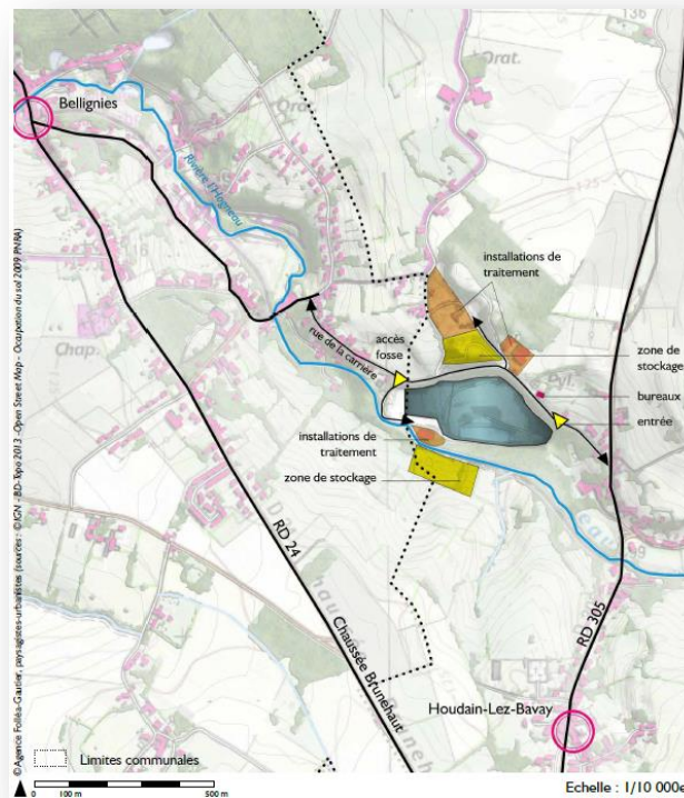
Figure 31 : Schéma de fonctionnement du site de Houdain-lez-Bavay.
