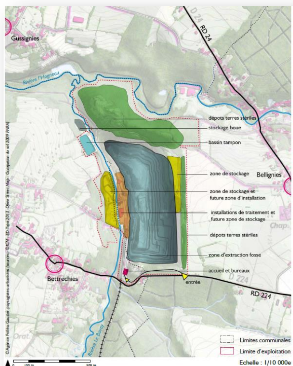
Figure 29 : Schéma de fonctionnement du site de Bellignies-Bettrechies.
