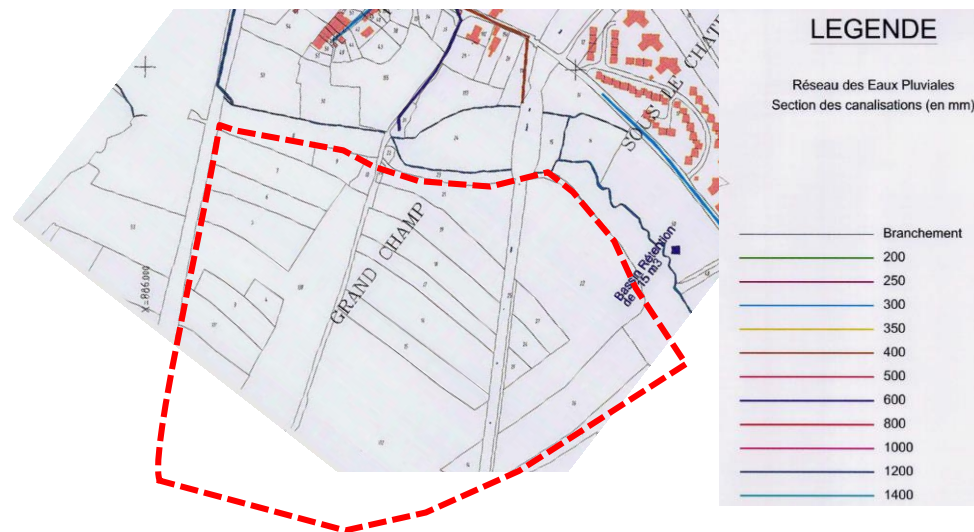
Réseau des eaux pluviales au droit du site d'étude
