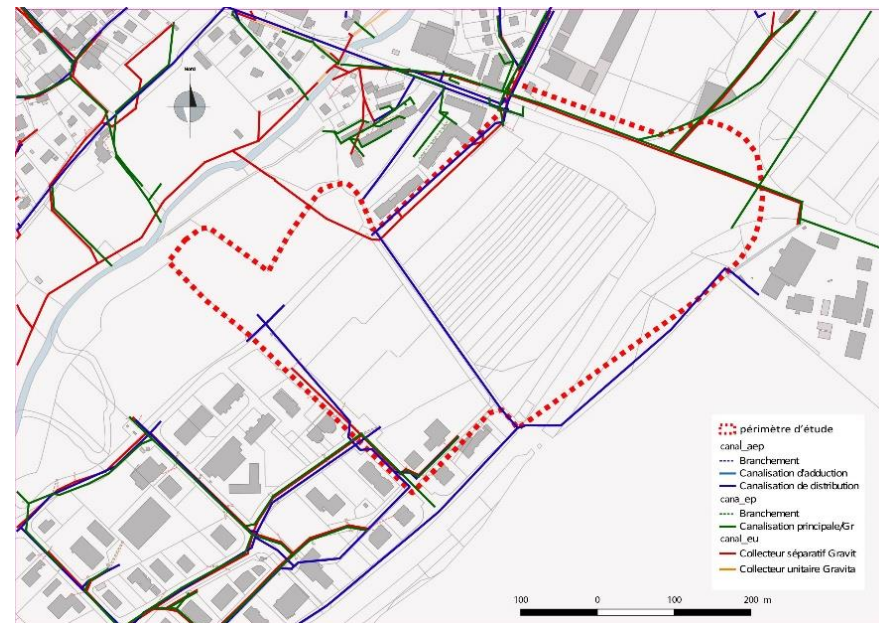
Desserte par les réseaux
