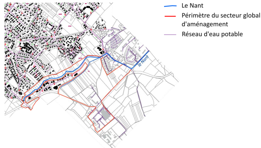
Réseau des eaux potables au droit du site d'étude
