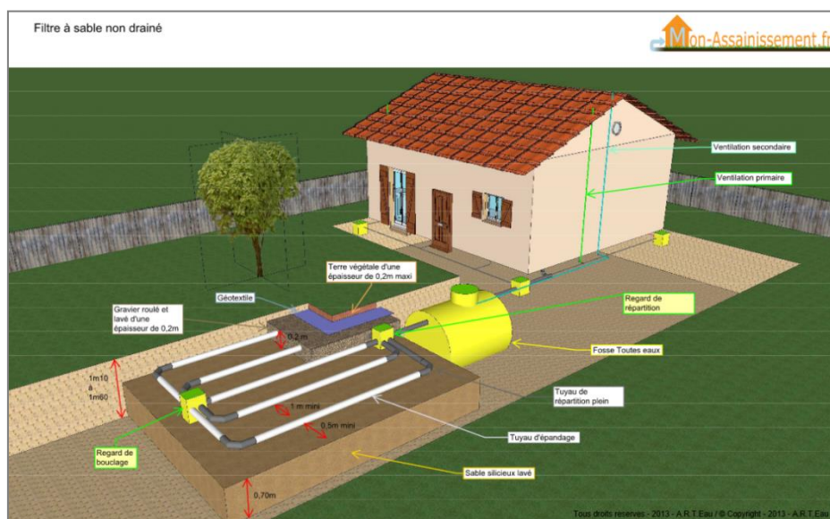
Figure 15 : Schéma d'un filtre à sable vertical non drainé (source : Mon-assainissement.fr)
