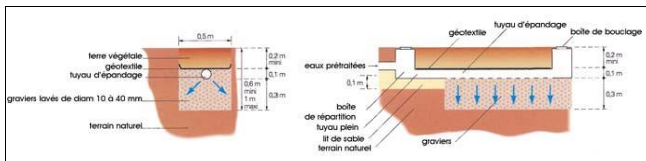
Figure 14 : Schéma d'une tranchée d'infiltration (source : Landrur.fr)
