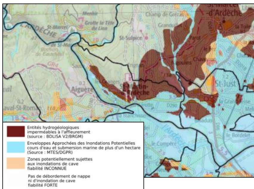
Figure 5 : Sensibilité aux remontées de nappe sur la commune de St Martin d'Ardèche (source : Infoterre)
