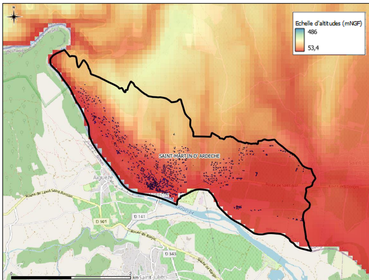
Figure 3 : Relief du territoire communal de St Martin d'Ardèche
