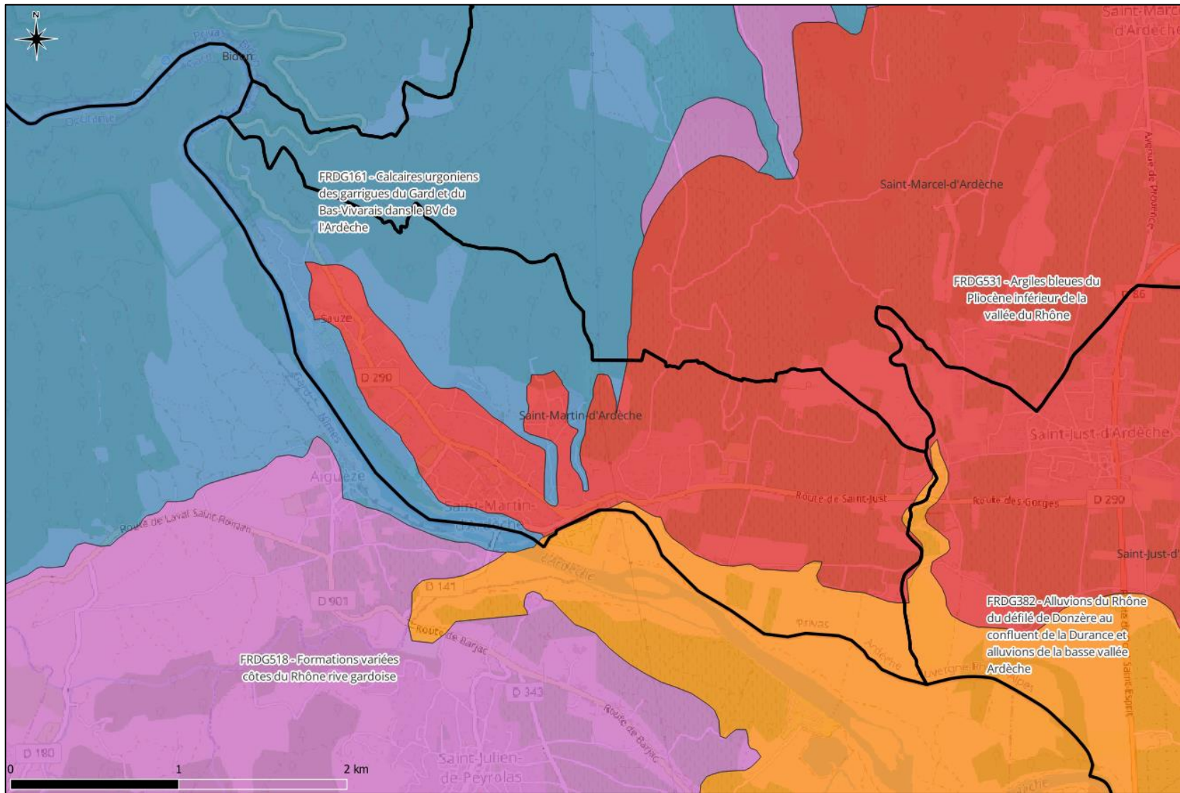
Figure 4 : Contexte hydrogéologique sur la commune de St Martin d'Ardèche (d'après données SDAGE 2022-2027)
