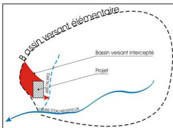
Figure 15 : Détermination du bassin versant intercepté
