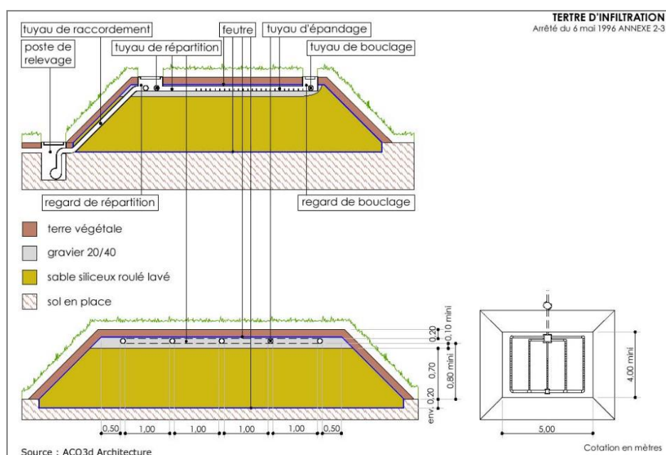
Figure 19 : Schéma d'un tertre d'infiltration (source : cc-hucqueliens.fr)
