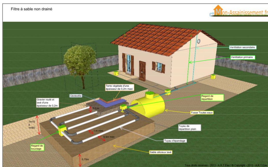
Figure 18 : Schéma d'un filtre à sable vertical non drainé (source : Mon-assainissement.fr)
