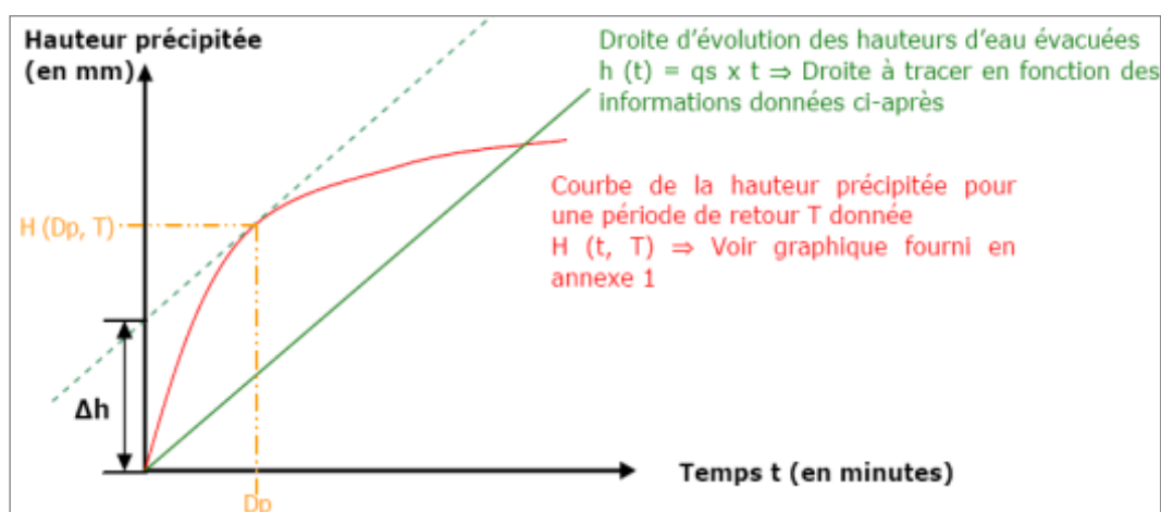
Figure 16 : Evolution de la hauteur d'eau précipitée et estimation par la méthode des pluies des hauteurs d'eau évacuées
