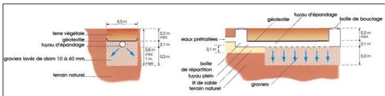
Figure 17 : Schéma d'une tranchée d'infiltration (source : Landrur.fr)
