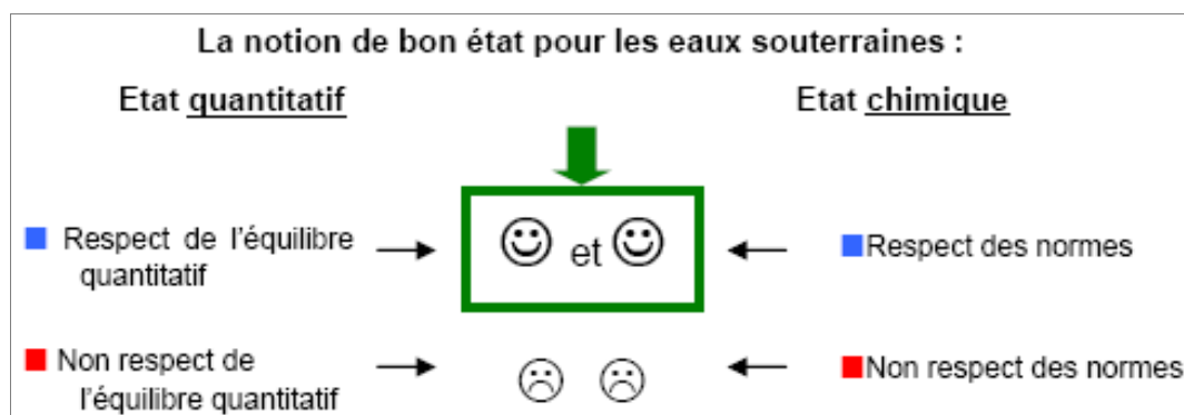
Figure 13 : Notion de bon état pour les eaux souterraines
