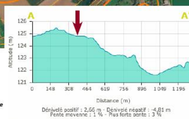
Coupes topographiques du secteur d'étude Source : www.geoportail.gouv.fr
