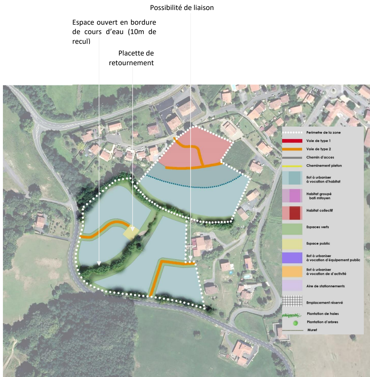
Fig. 7. Schéma d'aménagement du secteur 3
