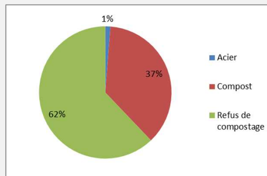
Performance de traitement de l'UVO pour 100kg OM traitées
