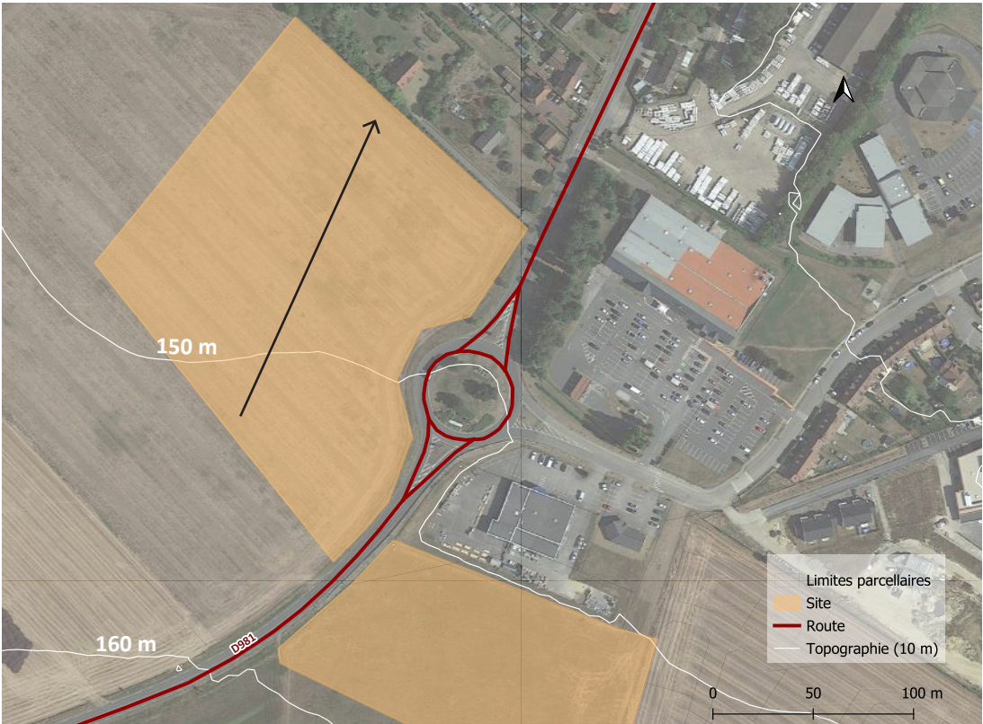
Axe de mesure de topographie- source : Oise MNT
