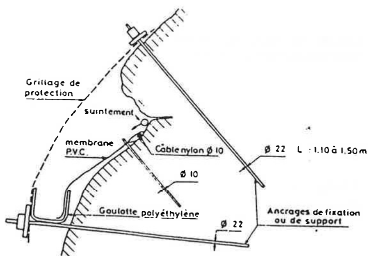
Exemple de dispositif de collecte en paroi
