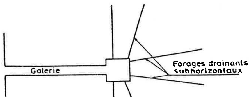
Schéma 3. galerie drainante associée à des forages drainants subhorizontaux ( vue en plan )
