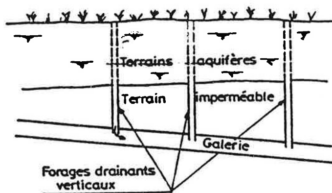
Schéma 2. galerie drainante associée à des forages drainants verticaux
