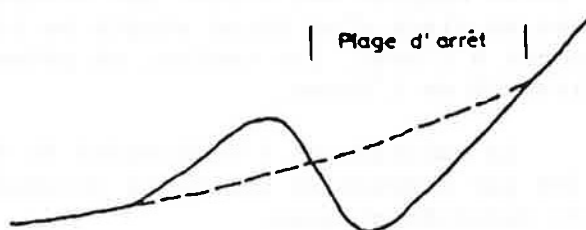
Plage d'arrêt constituée par un fossé associé à un écran massif
