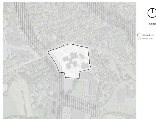
Carte 213 : OAP n°1 de Paimpol - Nuisance sonore
