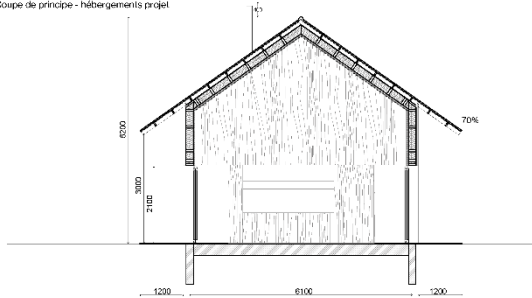
Coupe de principe - hébergements projet
