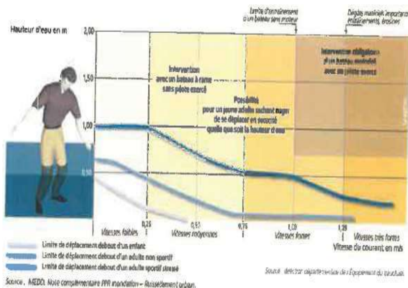
Illustration 6 : Capacité de déplacement d'un homme pendant une inondation
