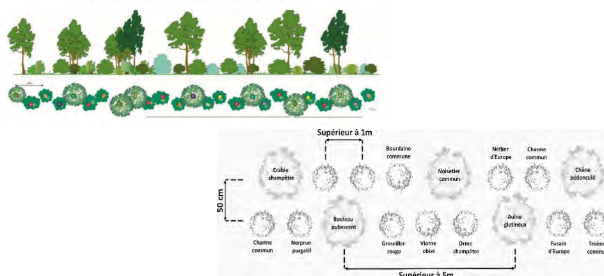
Figure 233 : exemples de haie multistrata (source : Écosphère)
