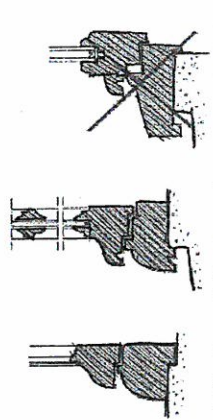
Profil ancien XIXe Profil contemporain proche de l'ancien Profil moderne inadapté
