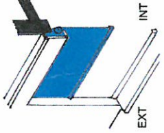
Caisson intégré à la devanture.
