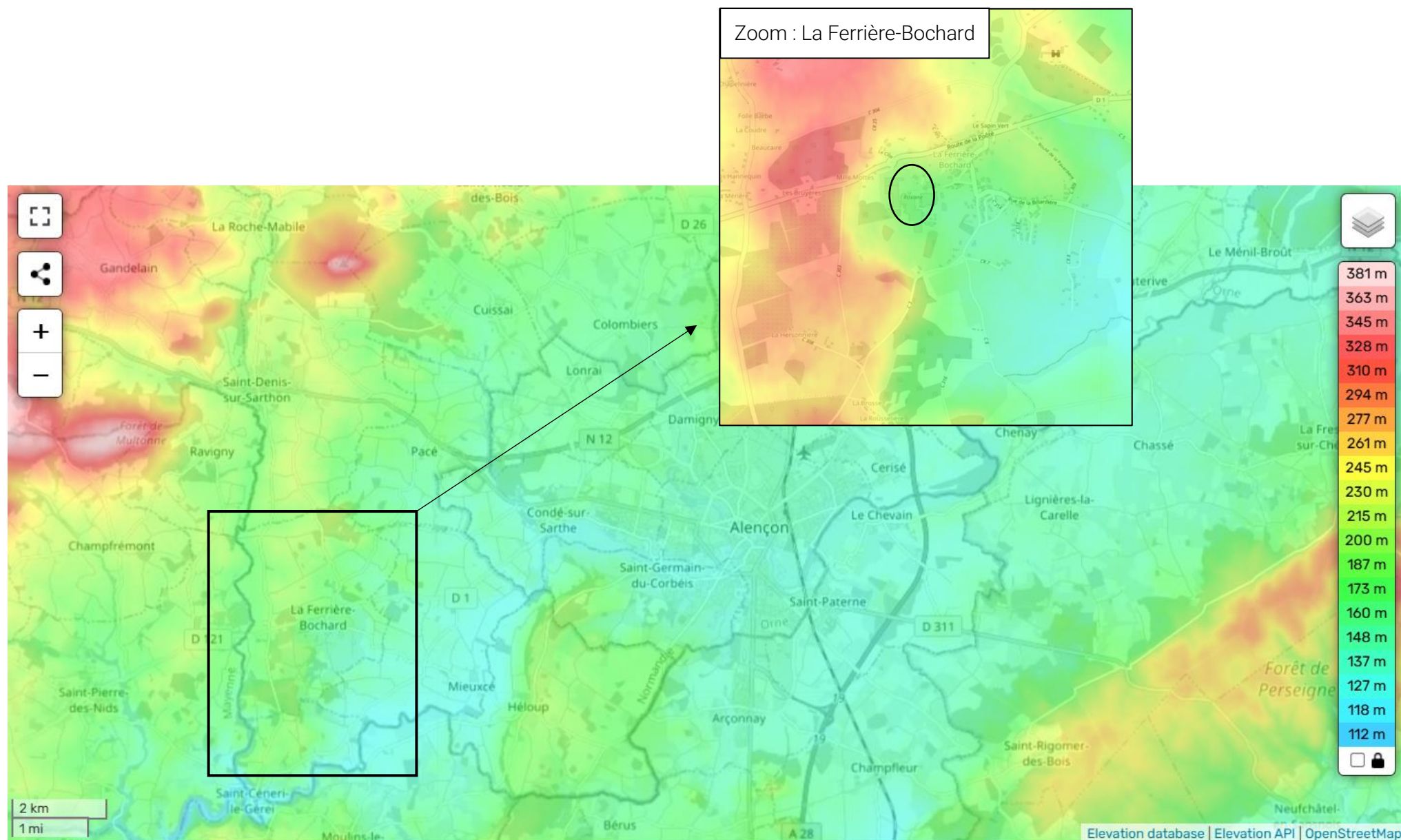
Figure 2 : Contexte topographique de la Communauté Urbaine d'Alençon, zoom sur la commune de la Ferrière-Bochard et le site de la révision allégée n°4 (Source : topographic-map.com ).
