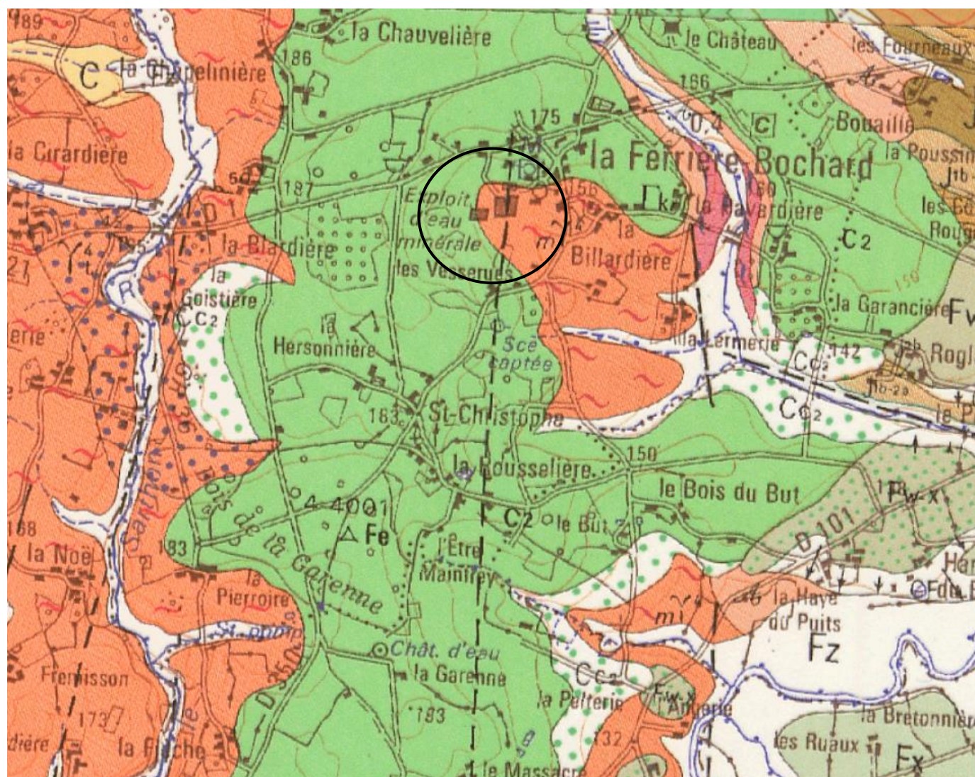
Figure 3 : Carte géologique 1/50 000 imprimé, zoom sur la commune de la Ferrière-Bochard et le site de la révision allégée n°4 (Source : SIGES Seine-Normandie )
