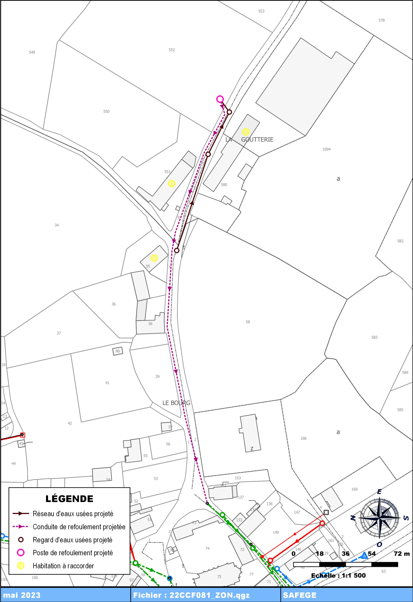
Figure n°10 : Commune de Arpheuilles-Saint-Priest - Scénario d'aménagement collectif – Secteur Rue de la Croix du Chiez
