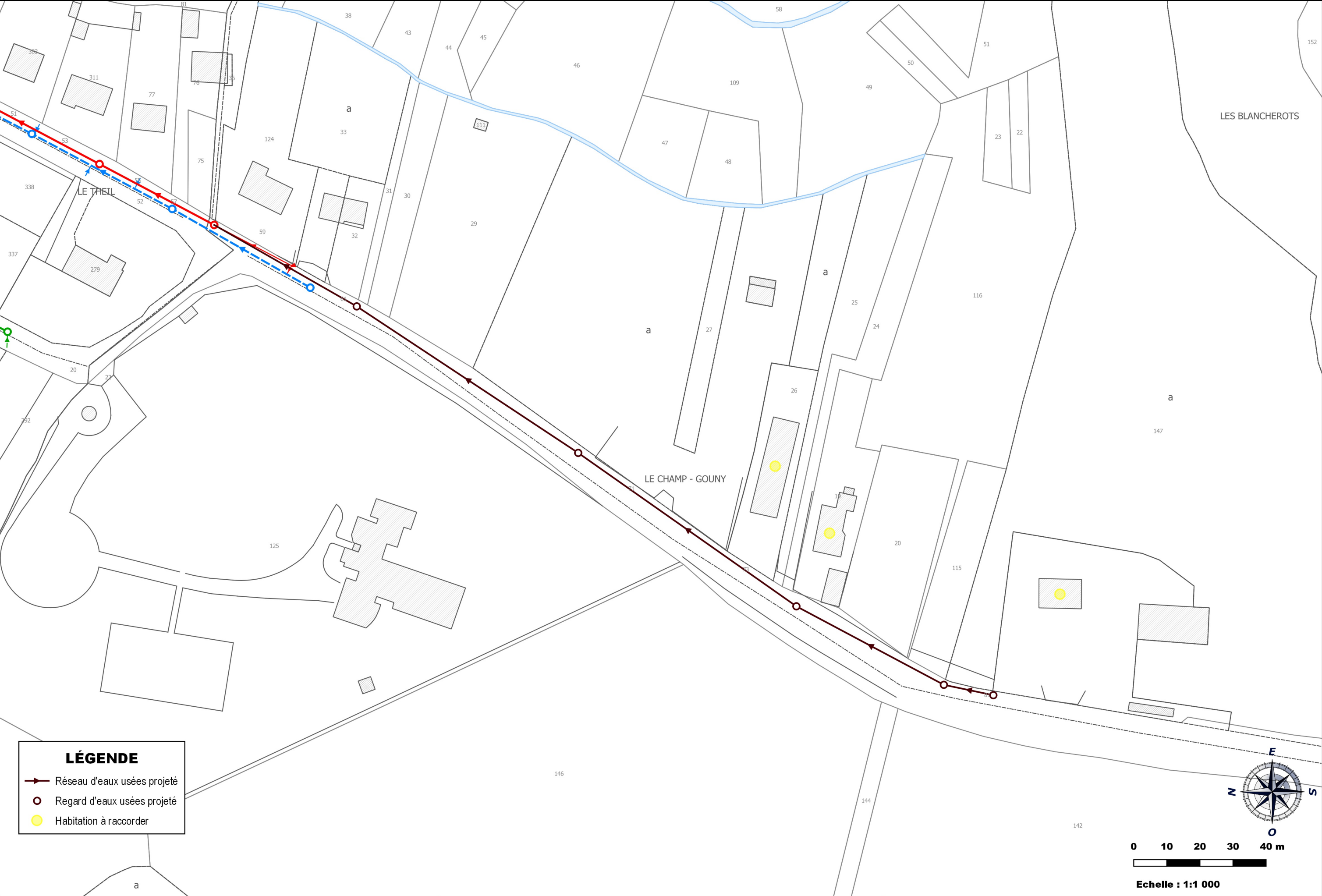
Figure n°10 : Commune de Lavault-Sainte-Anne - Scénario d'aménagement collectif – Secteur RD 304 - Le Theil
