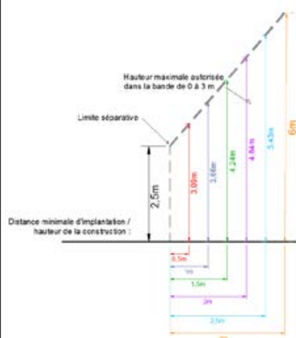
Gabarit opposable pour la bande de 0 à 3 m
