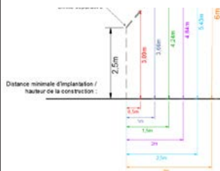
Gabarit opposable pour la bande de 0 à 3 m
