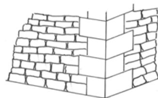
Schéma d'un chaînage d'angle (source : CAUE Franche-Comté)
