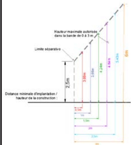
Gabarit opposable pour la bande de 0 à 3 m
