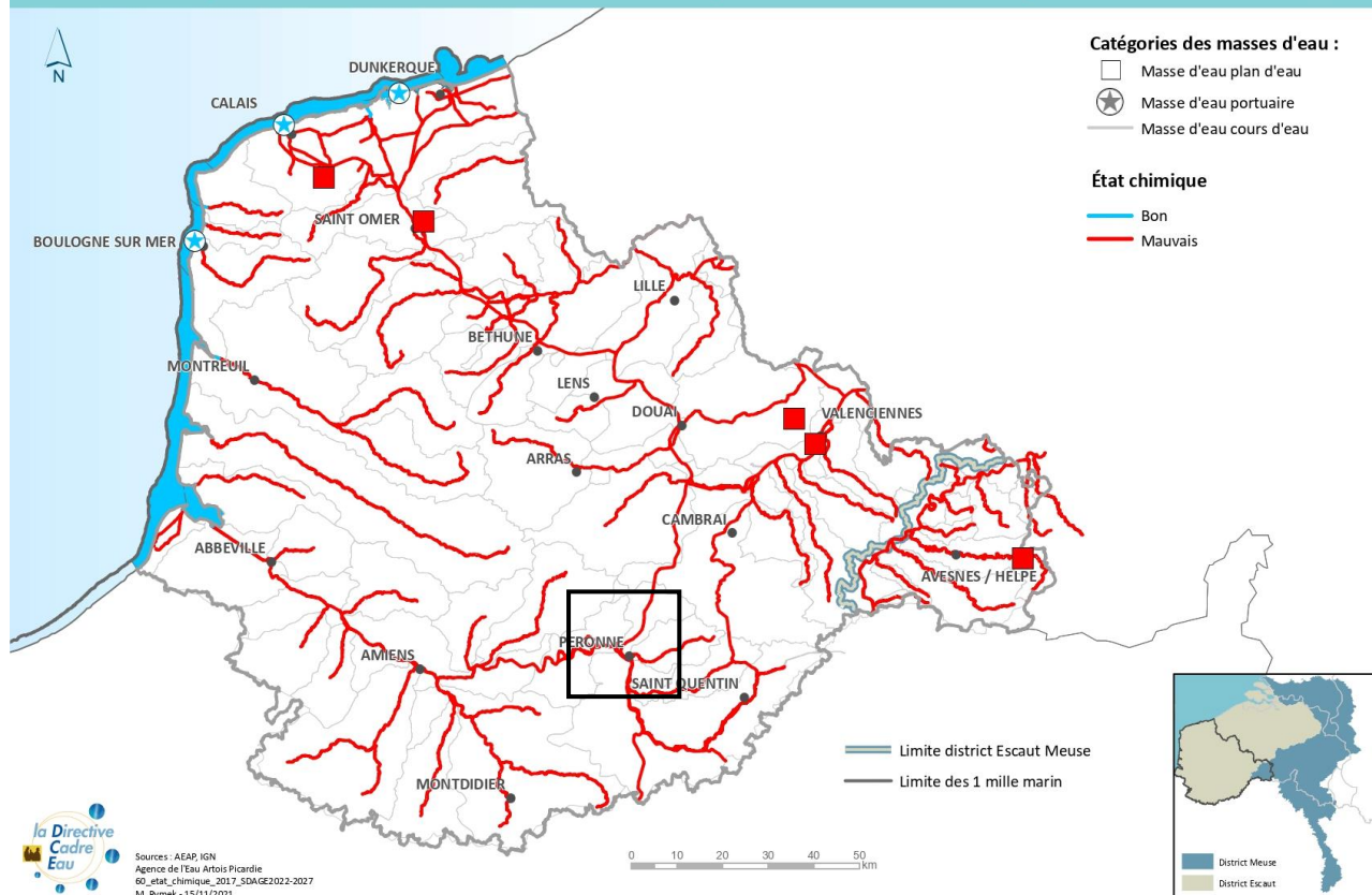
Etat chimique des eaux de surface 2015-2017 – Agence de l'Eau Artois Picardie
