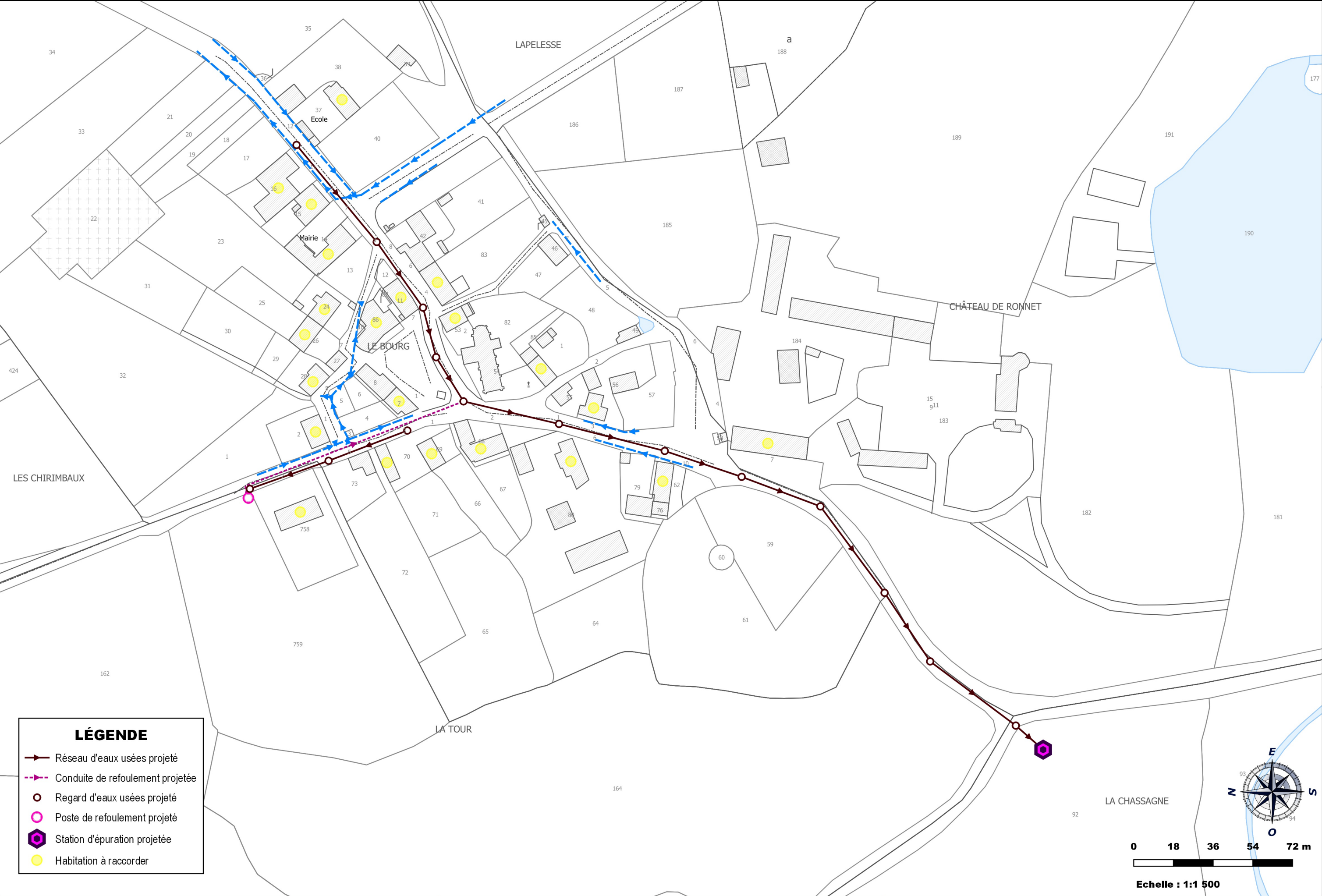
Figure n°10 : Commune de Ronnet - Scénario d'aménagement collectif – Secteur du Bourg
