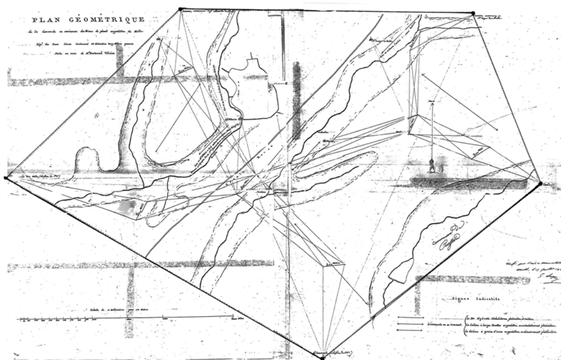
Figure 14 - Plan de la demande en concession des mines de plomb argentifère de Melle faite au nom de M. Bertrand Villain (arch. Société d'Archéologie et de Spéléologie du Mellois, comm. F. Tereygeol, 2009).
