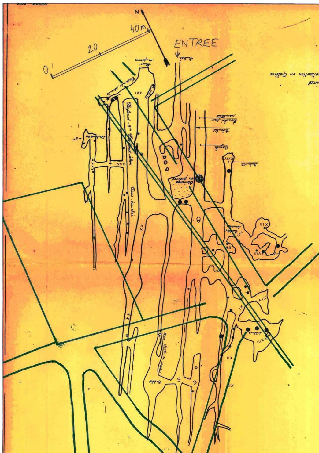
Figure 39 - Travaux G7 de la Rue des Mines : plan levé le 19 novembre et les 3 et 10 décembre 1944 à 1/400, annexé au rapport BRGM de 1959.
