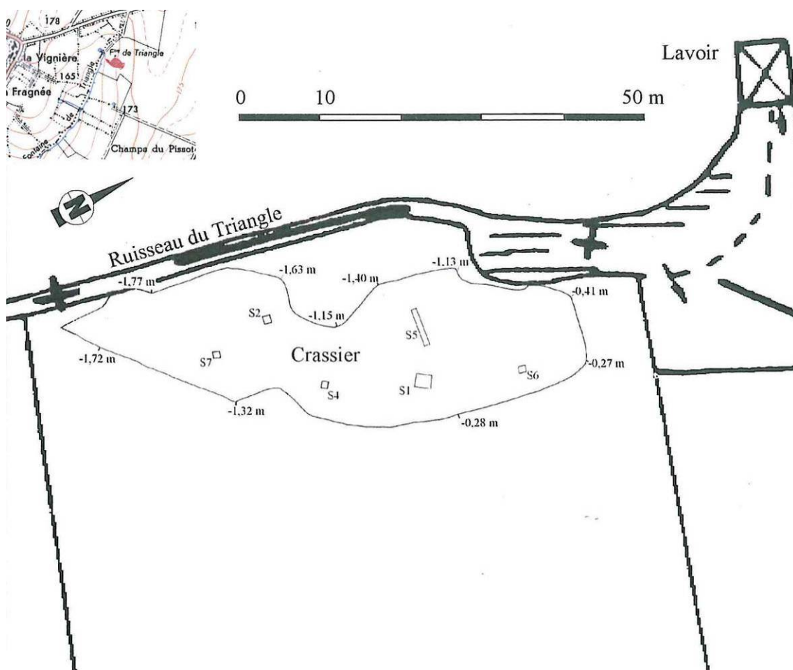
Figure 27 - Carte du crassier de la Fontaine du Triangle (Tereygeol, 2001).
