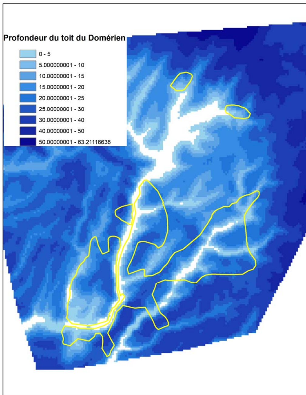
Figure 52 - Profondeur du toit du Domérien (en m) par rapport à l'emprise des travaux.
