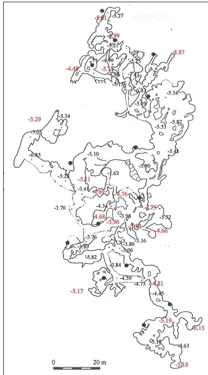
Figure 44 - Plan du réseau TDF (P3) avec cote relative (Tereygeol, 2001). En rouge, de points topo pris sur le rocher et, en noir, de points topo pris sur les remblais ; mesures en mètres à partir de la plaque métallique d'accès.
