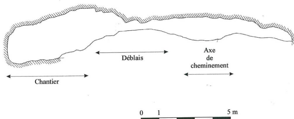
Figure 19 - Coupe type d'une chambre avec front d'abattage au feu dans le réseau TDF (Tereygeol, 2001).
