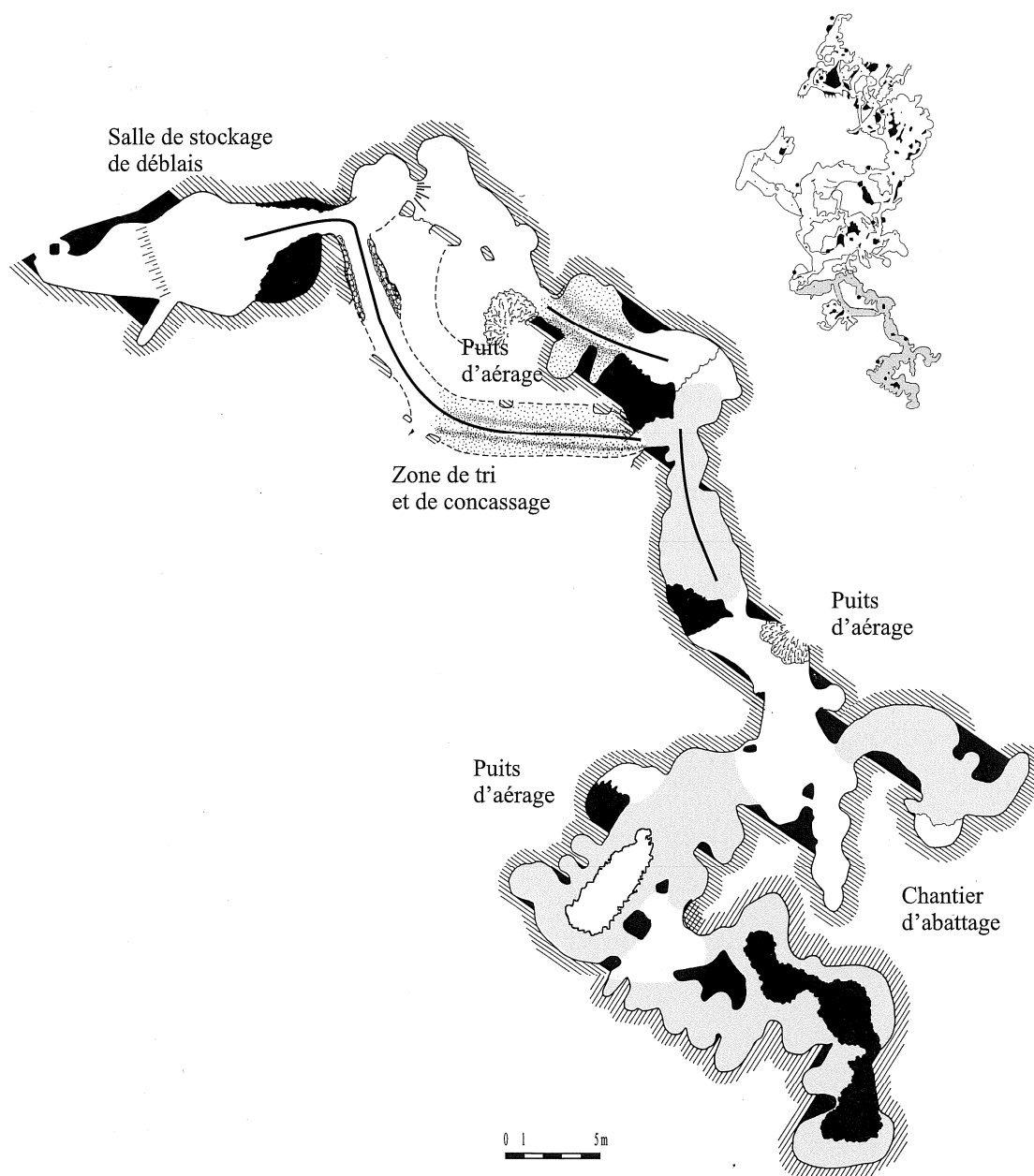
Figure 15 - Plan de la partie sud du réseau TDF (ouvrage P3) montrant l'allure des chambres de creusement au feu (Tereygeol, 2001).
