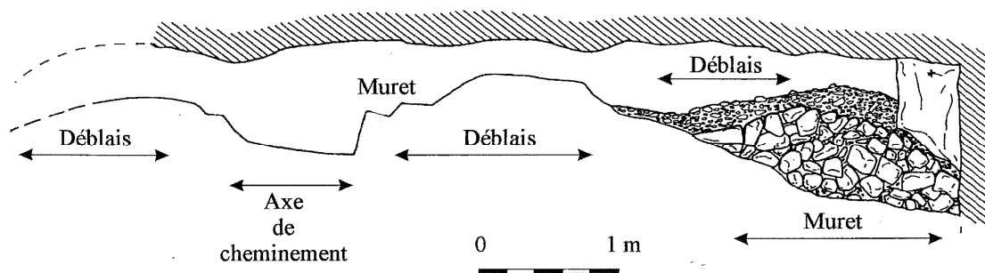
Figure 20 - Coupe type d'une ancienne chambre d'abattage dans le réseau TDF, avec remblais et axe de cheminement (Tereygeol, 2001).
