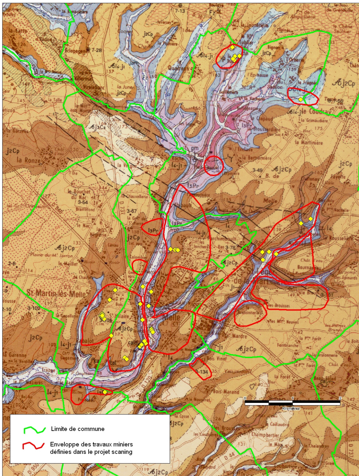
Figure 2 - Carte géologique (extraite des feuilles Melle et Saint-Maixent à 1/50 000) avec les éléments de la figure précédente.
