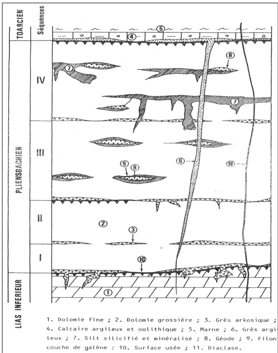
Figure 6 - Coupe type du Pliensbachien de Melle (S. Coiteux, 1982) montrant la minéralisation en filons-couches et géodes de carbonates à cristaux de galène dans les séquences III et IV.
