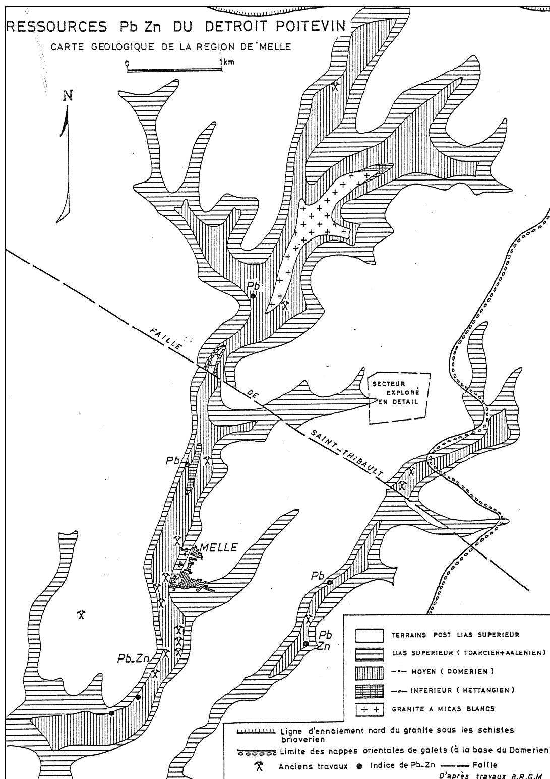
Figure 4 - Carte géologique schématique des boutonnières de la Béronne et de la Légère.
