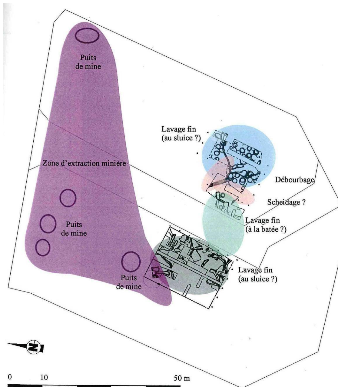
Figure 24 - Organisation des espaces dans la laverie des Boulitotes (Tereygeol, 2001).
