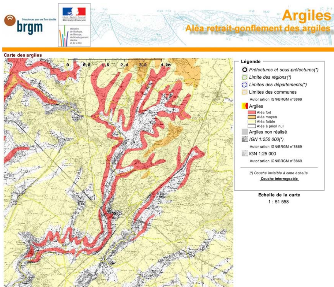
Figure 54 - Carte d'aléa retrait gonflement sur la commune de Melle.
