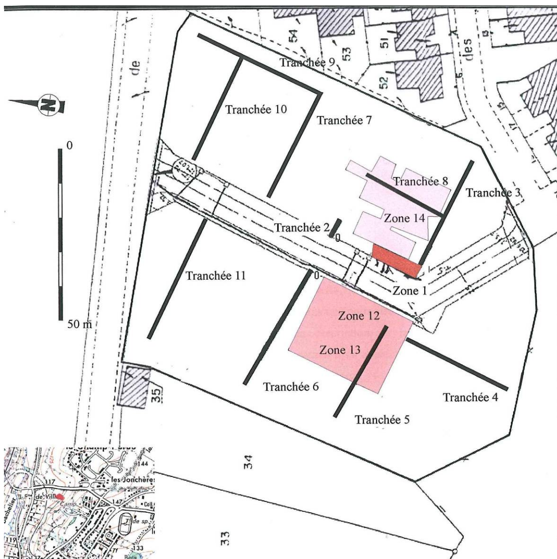
Figure 25 - Plan de la laverie des Boulitotes (Tereygeol, 2001).
