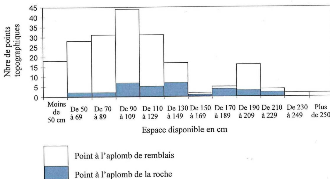
Figure 21 - Histogramme de la hauteur actuelle des chambres dans le réseau TDF, hauteur sur roche ou hauteur sur remblai (Tereygeol, 2001).
