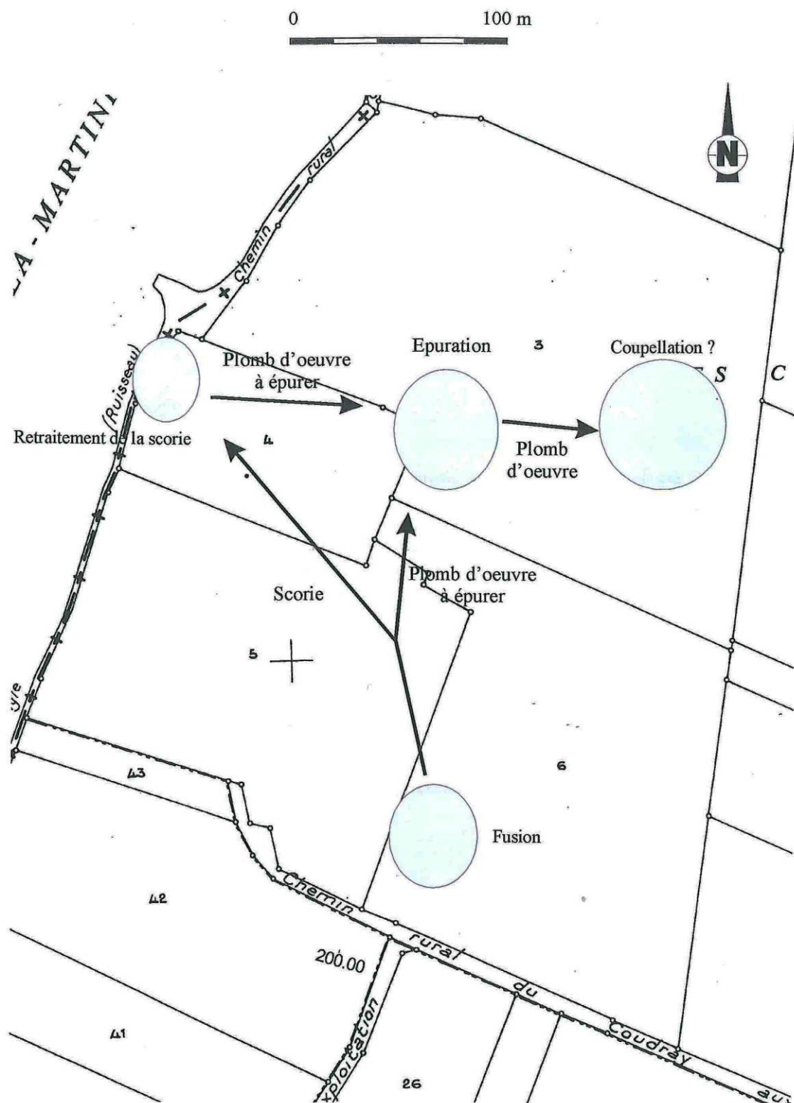
Figure 26 - Organisation des espaces à la fonderie de la Fontaine du Triangle (Tereygeol, 2001).
