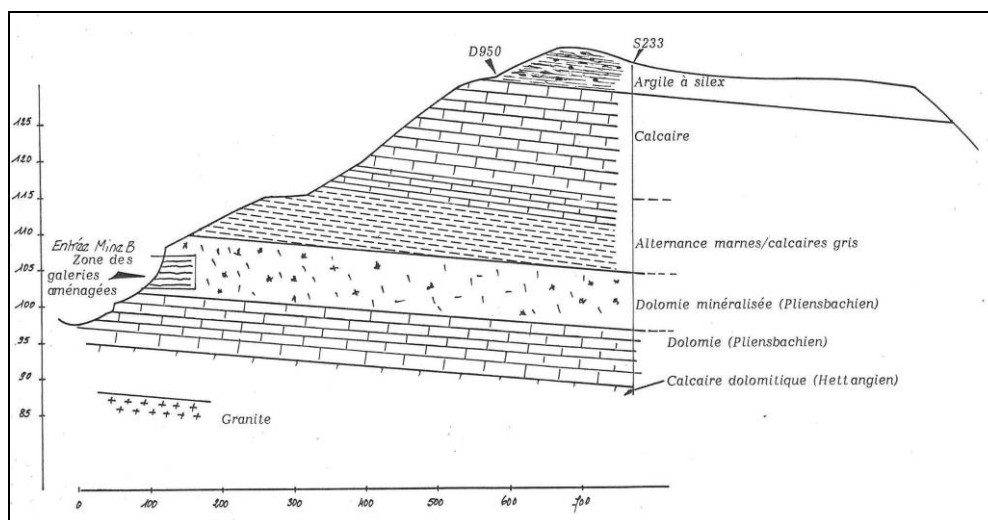
Figure 29 - Coupe géologique de la mine aménagée du Jardinier (Both, 1987).
