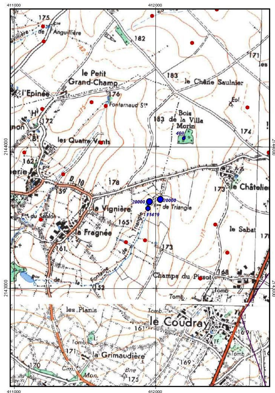
Figure 28 - Carte du secteur de la fonderie de la Fontaine du Triangle montrant l'intensité de la pollution au plomb (BRGM, A. Lambert, 2002).
