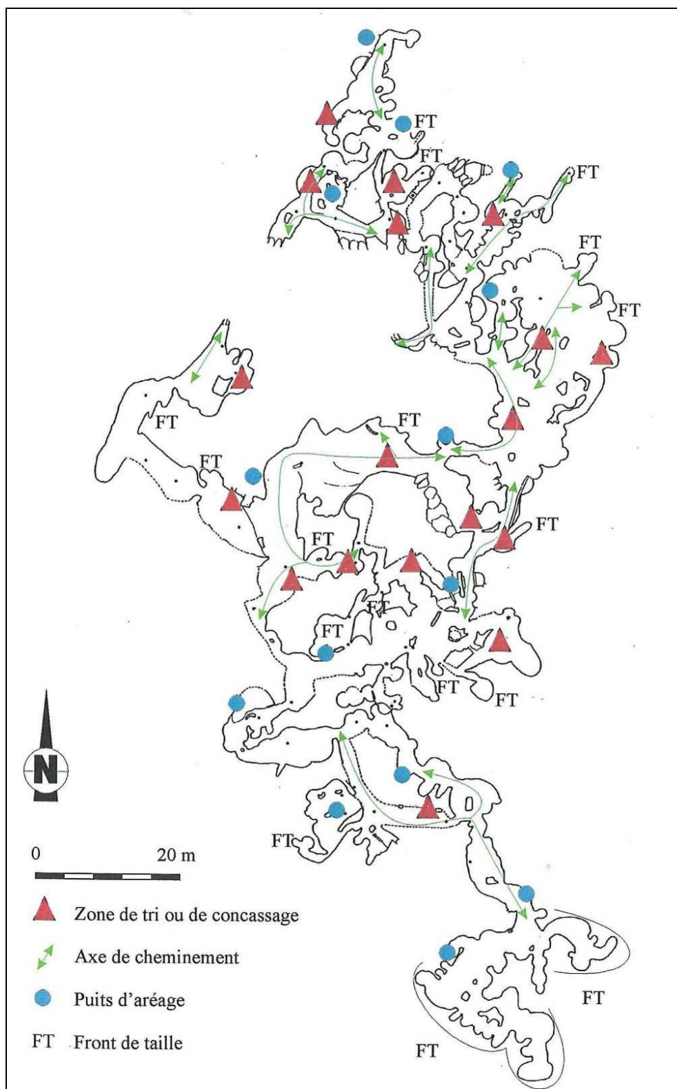
Figure 43 - Plan du réseau TDF (P3) (Tereygeol, 2001).
