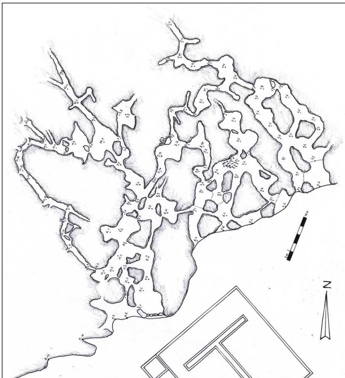
Figure 37 - L'Araignée : plan du spéléo-club du Pays Mellois (levé J.-L. Denis et coll.).
