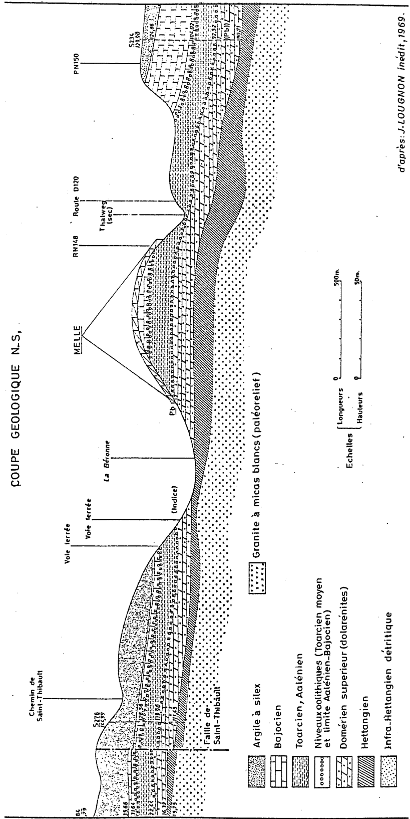
Figure 8 - Coupe de détail nord-sud à travers la partie centrale du gisement. Rappel : la minéralisation affecte la moitié supérieure du Domérien (Pliensbachien), au mur des marnes du Toarcien
