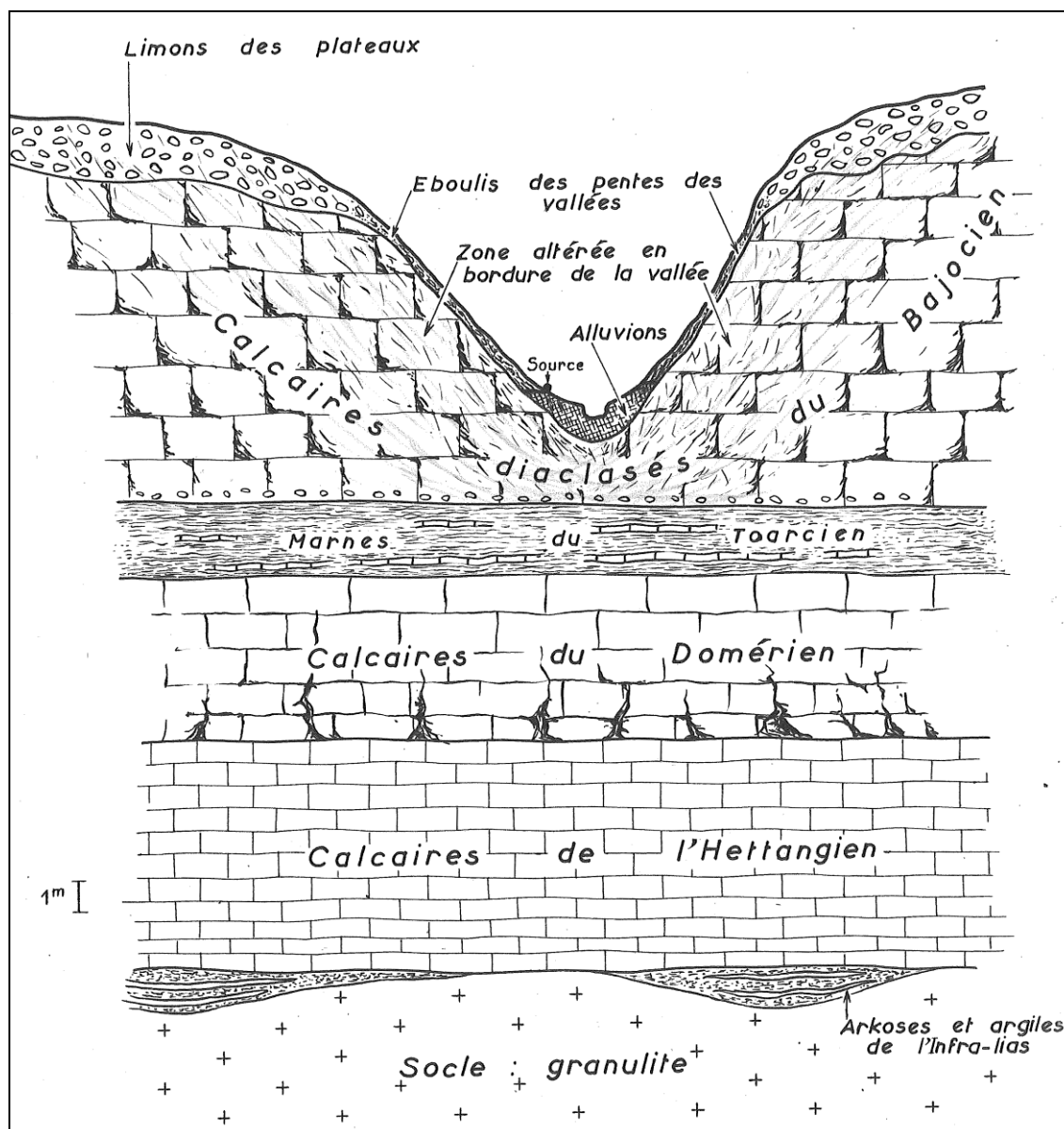
Figure 5 - Coupe schématique du Lias à Melle (la minéralisation affecte la moitié supérieure des calcaires du Domérien).
