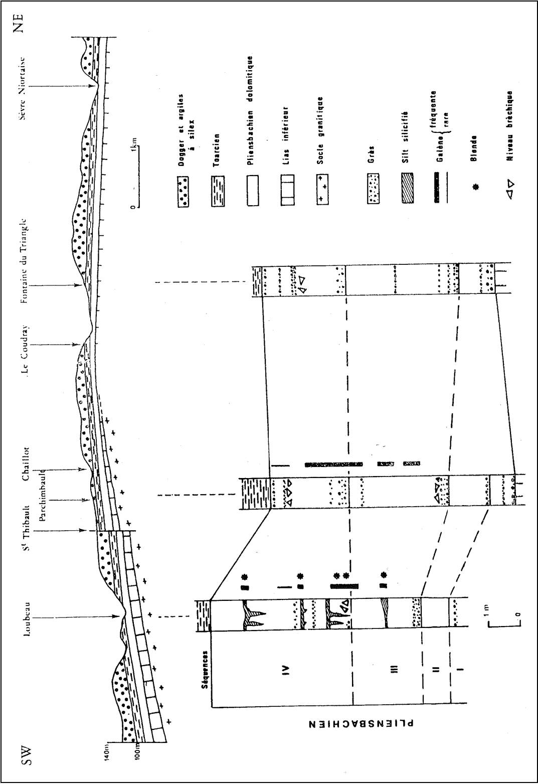
Figure 10 - Variation latérale de l'intensité de la karstification et de la minéralisation, d'après S. Coiteux (1982).
