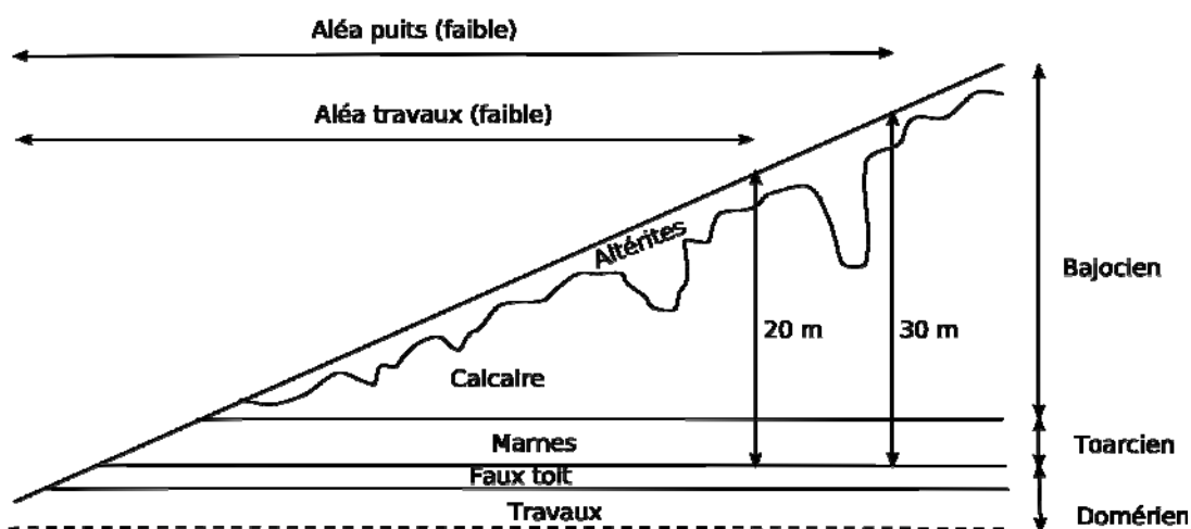
Figure 57 - Schématisation de la détermination des zones d'aléa effondrement localisé sur puits et sur travaux.
