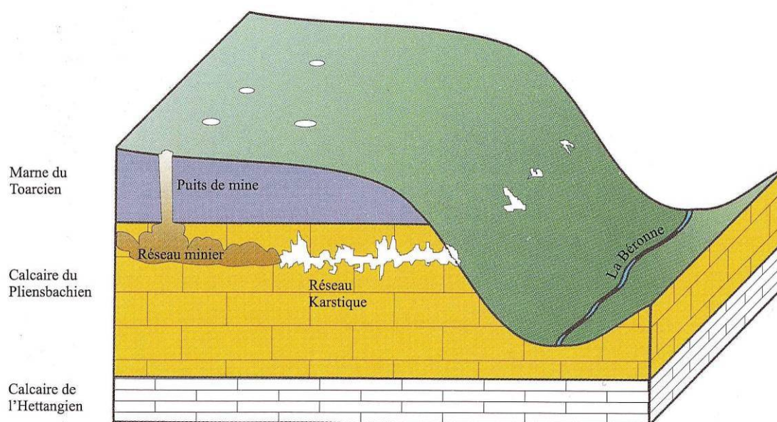
Figure 17 - Bloc diagramme montrant la localisation des puits par rapport aux chambres d'exploitation et le passage d'un réseau minier au réseau karstique vierge impénétrable aux hommes de la taille d'aujourd'hui (Tereygeol, 1999).
